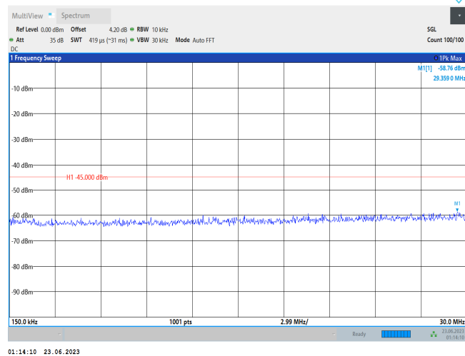
Band7-20MHz-QPSK-20850-1RB#0-Range2:0.15~30MHz
