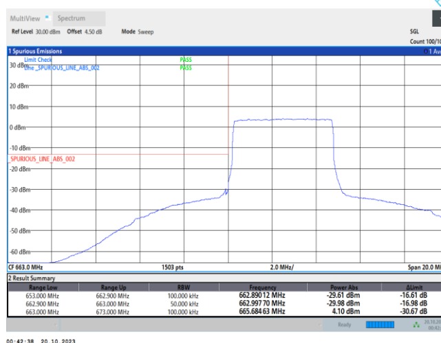
Band71-5MHz-QPSK-133147-25RB#0
