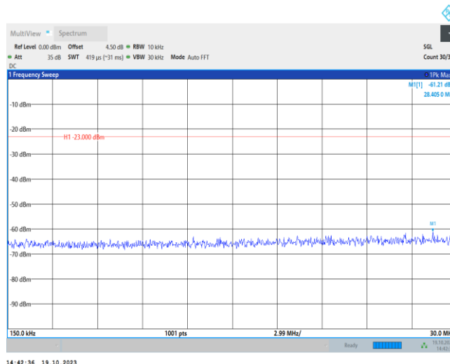
Band13-10MHz-QPSK-23230-1RB#0-Range2:0.15~30MHz
