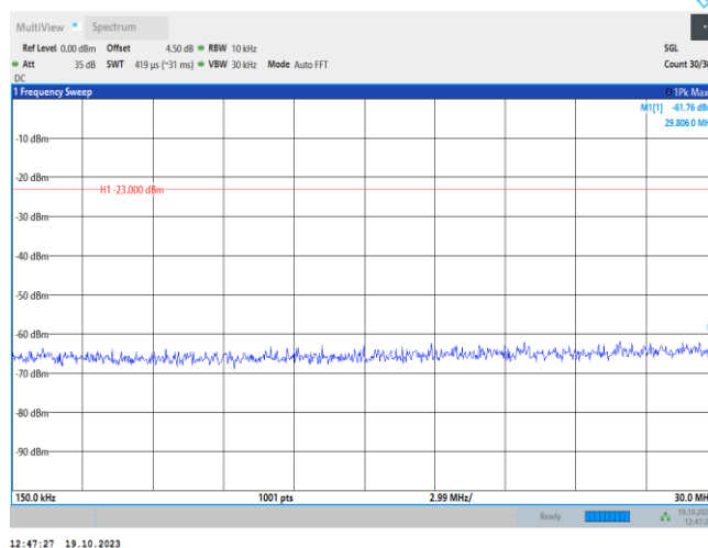
Band12-10MHz-QPSK-23060-1RB#0-Range2:0.15~30MHz
