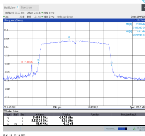
11ac80SISO-Ant9-5530
