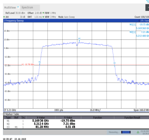
11ac80SISO-Ant9-5210
