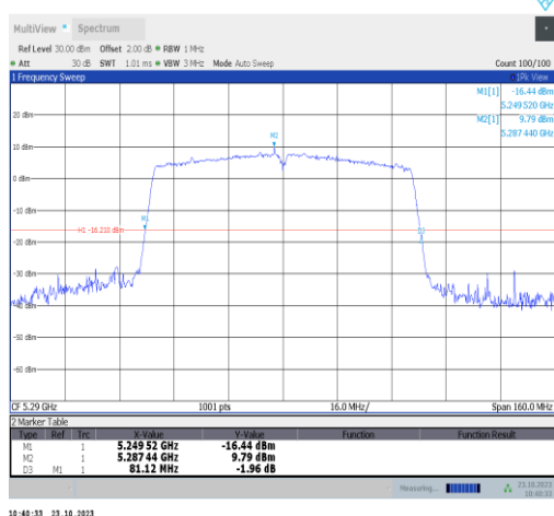
11ac80SISO-Ant9-5290
