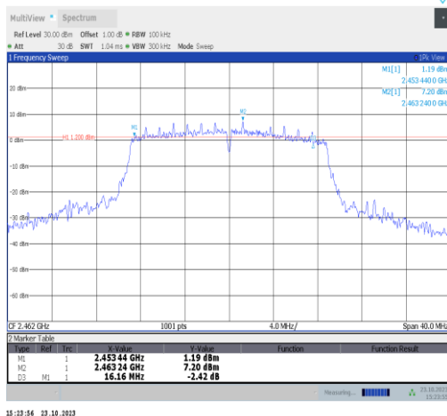
11n20ISO-Ant9-2462-PASS
