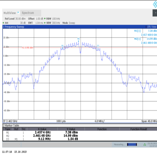
11b-Ant9-2462-PASS
