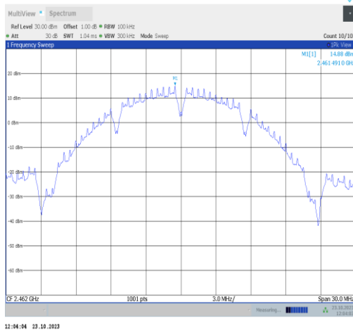
11b-Ant9-2462-0~Reference-PASS
