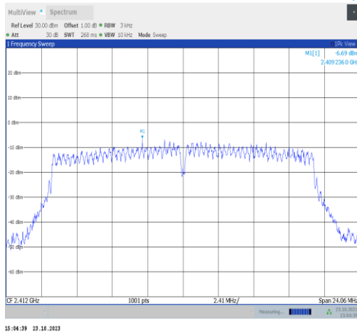
11n20ISO-Ant9-2412-PASS
