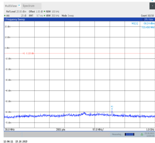
11b-Ant9-2462-30~1000-PASS
