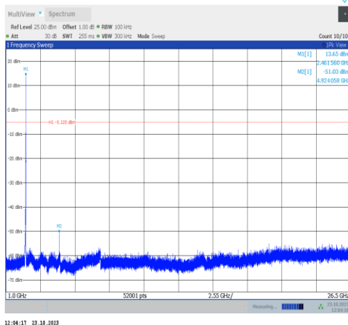
11b-Ant9-2462-1000~26500-PASS
