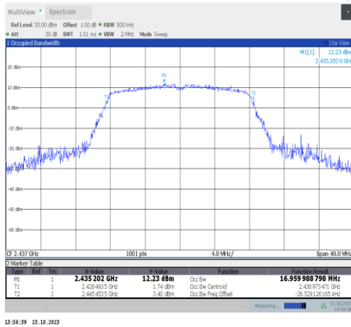
11g-Ant9-2437
