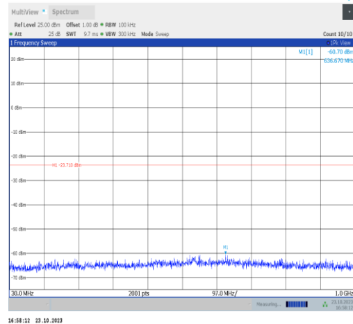
BLE_2M-Ant9-2440-30~1000-PASS
