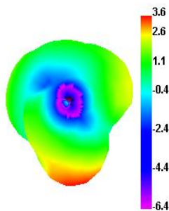
2450.000MHz
