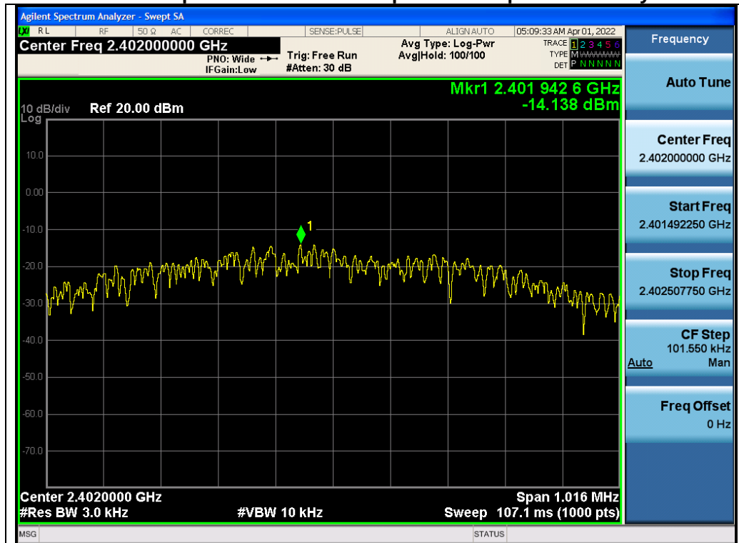
Test_Graph_LE1M_ANT2_2402_1Mbps_PSD
