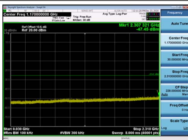
,Plot 3,30MHz~2310MHz-802.11n(HT40) ,2437MHz
