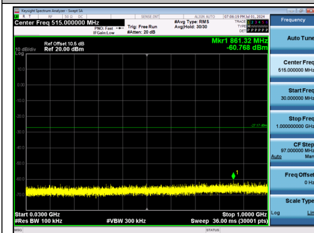
11G-Ant1-2462-30~1000-PASS
