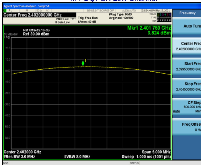
\pi/4 -DQPSK Low Channel
