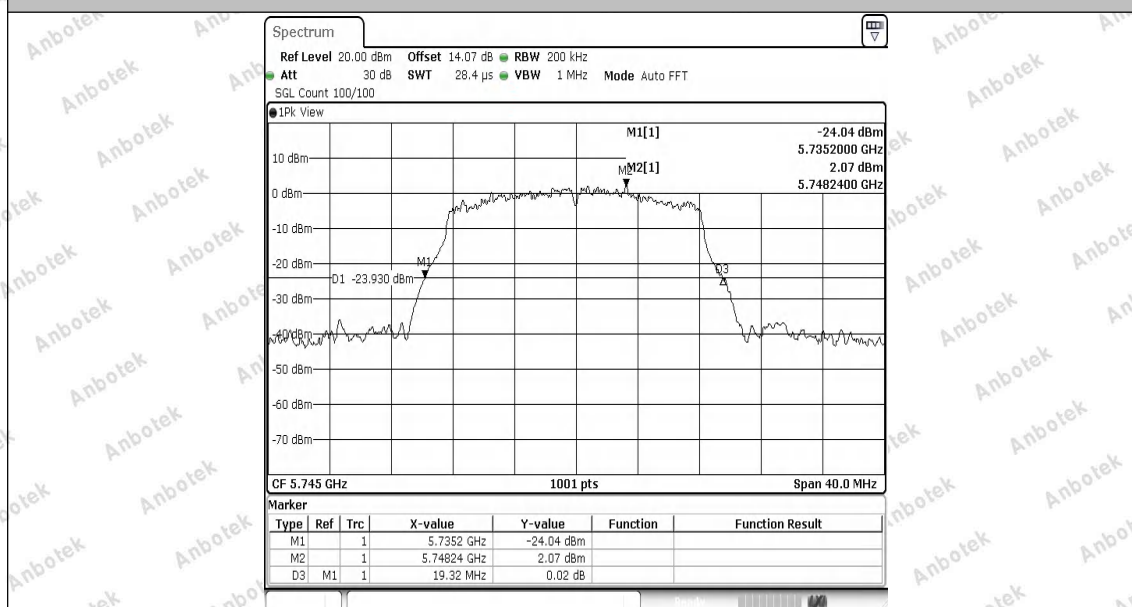
11A-Ant1-5745
