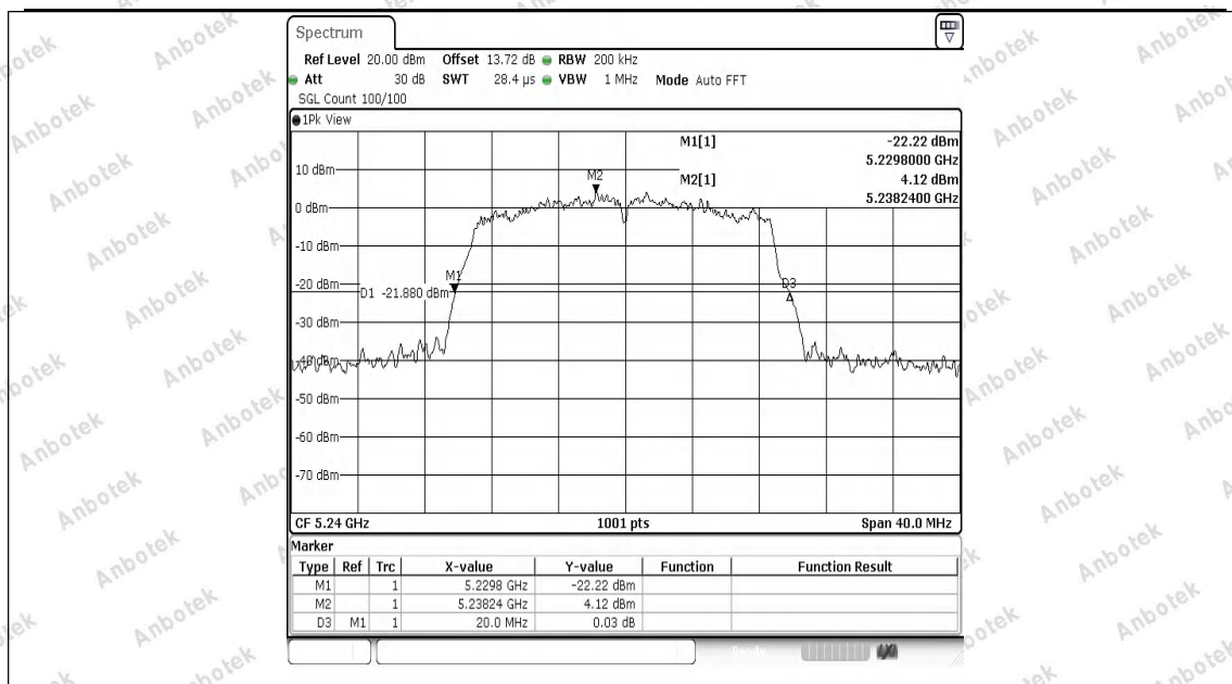
11N20MIMO-Ant1-5240
