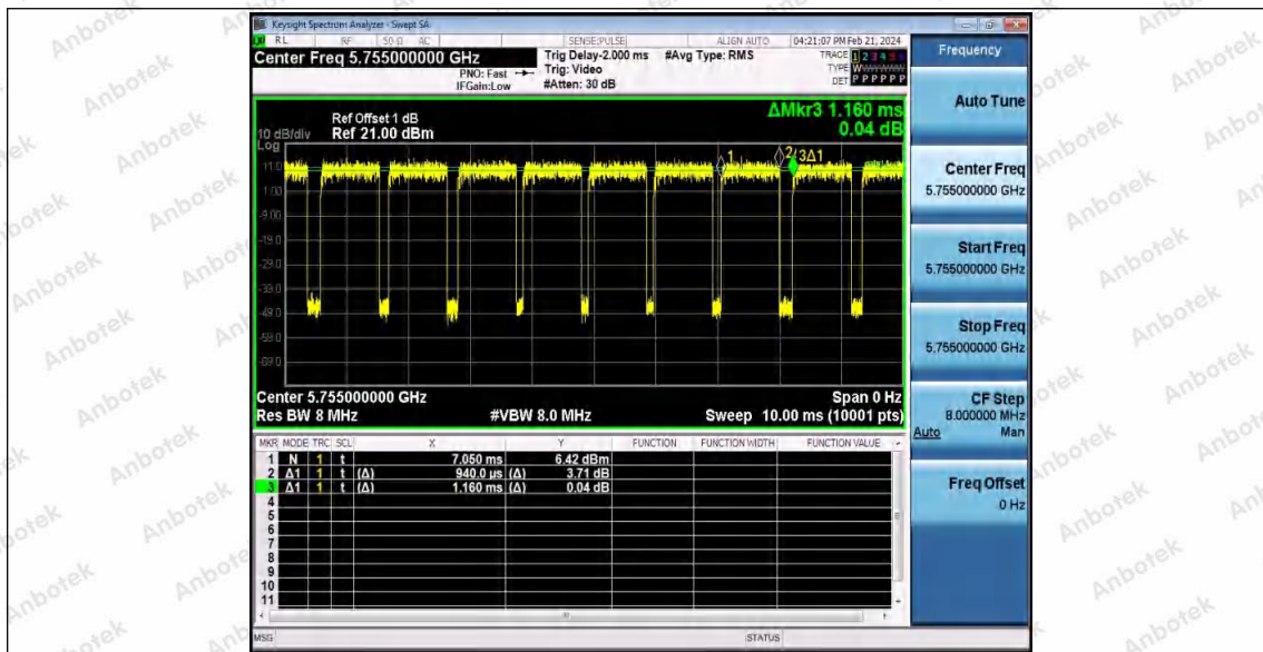
11AC40MIMO_Ant2_5755
