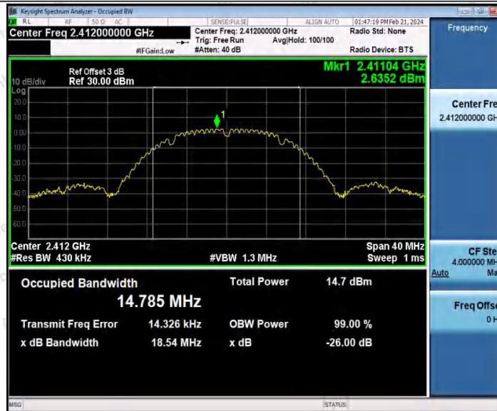
11B-CDD_Ant2_2412
