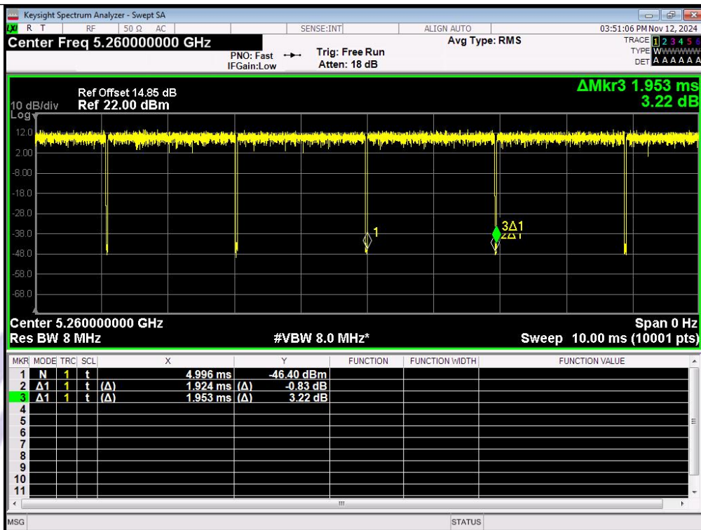
IEEE 802.11n_20MHz_Channel 52
