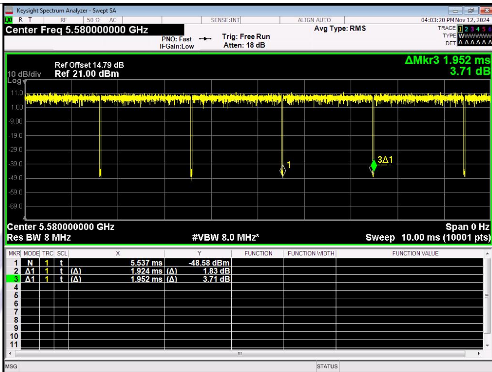
IEEE 802.11n_20MHz_Channel 116
