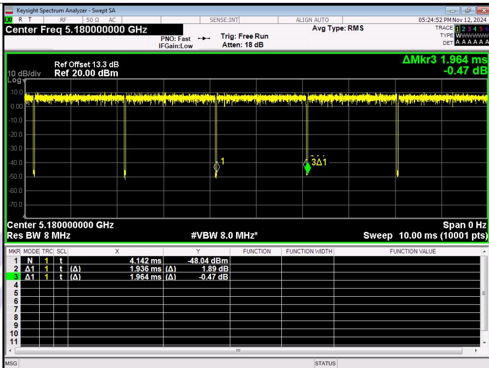
IEEE 802.11ac_20MHz_Channel 36
