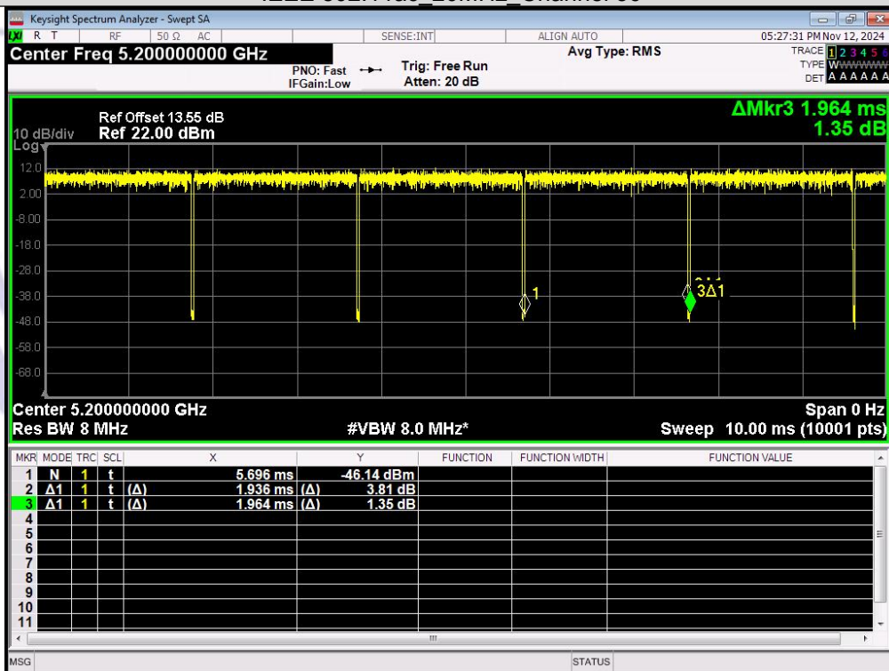
IEEE 802.11ac_20MHz_Channel 40
