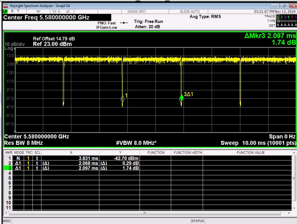
IEEE 802.11a_20MHz_Channel 116
