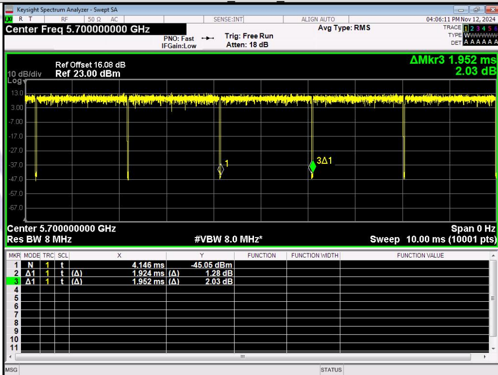
IEEE 802.11n_20MHz_Channel 140
