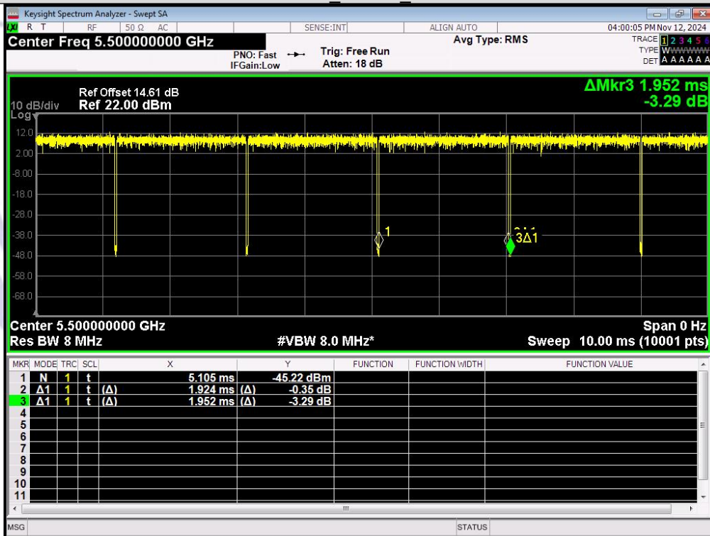
IEEE 802.11n_20MHz_Channel 100
