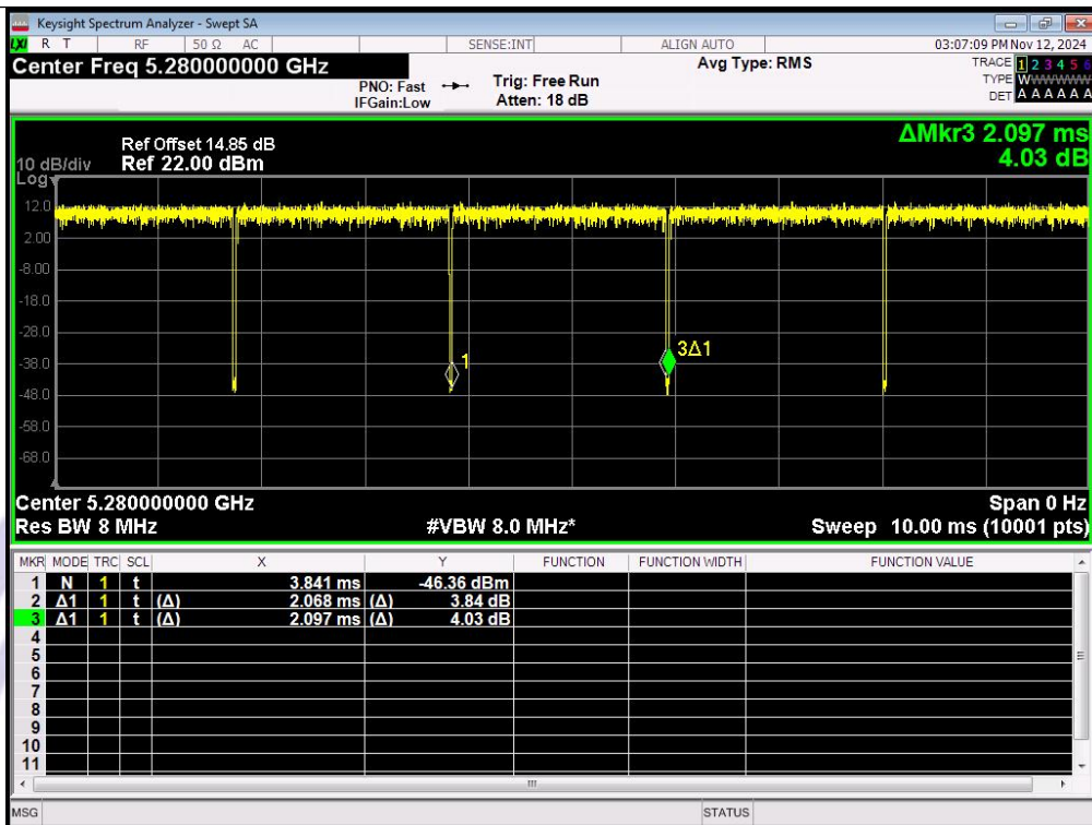
IEEE 802.11a_20MHz_Channel 56
