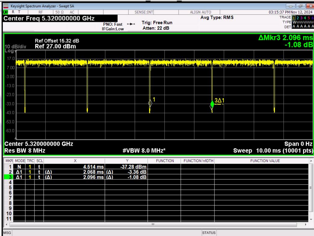
IEEE 802.11a_20MHz_Channel 64
