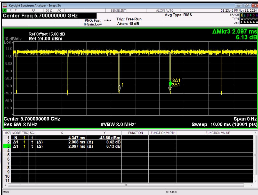
IEEE 802.11a_20MHz_Channel 140
