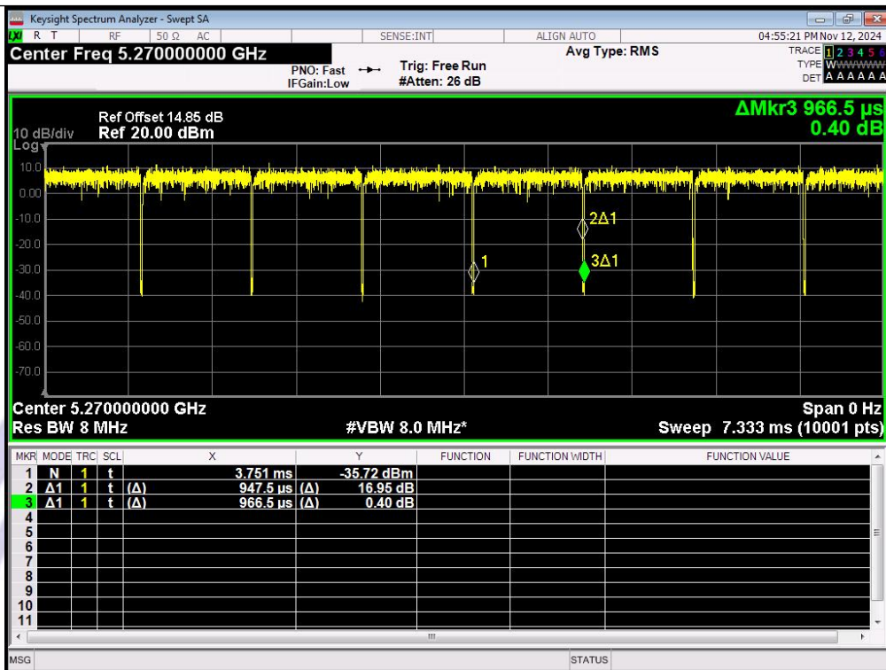
IEEE 802.11n_40MHz_Channel 54
