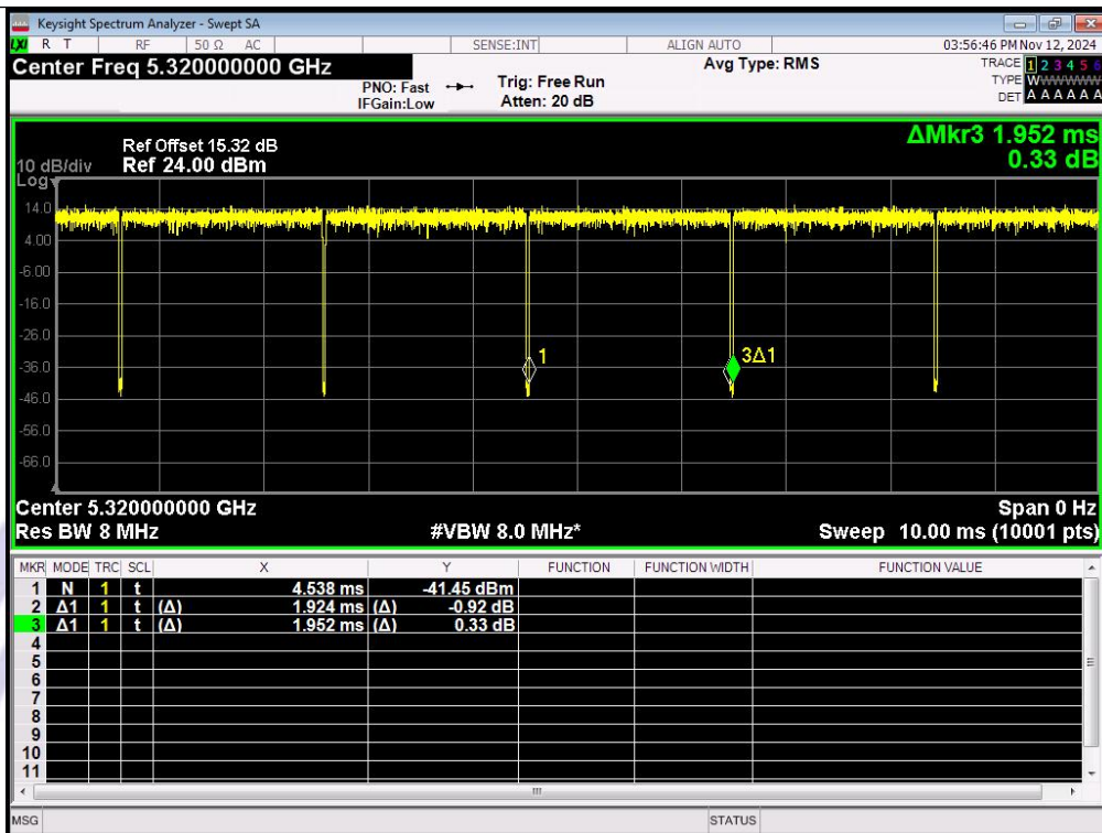
IEEE 802.11n_20MHz_Channel 64
