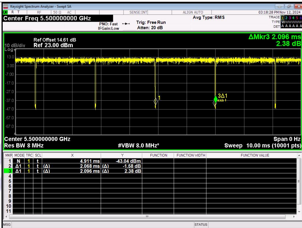
IEEE 802.11a_20MHz_Channel 100
