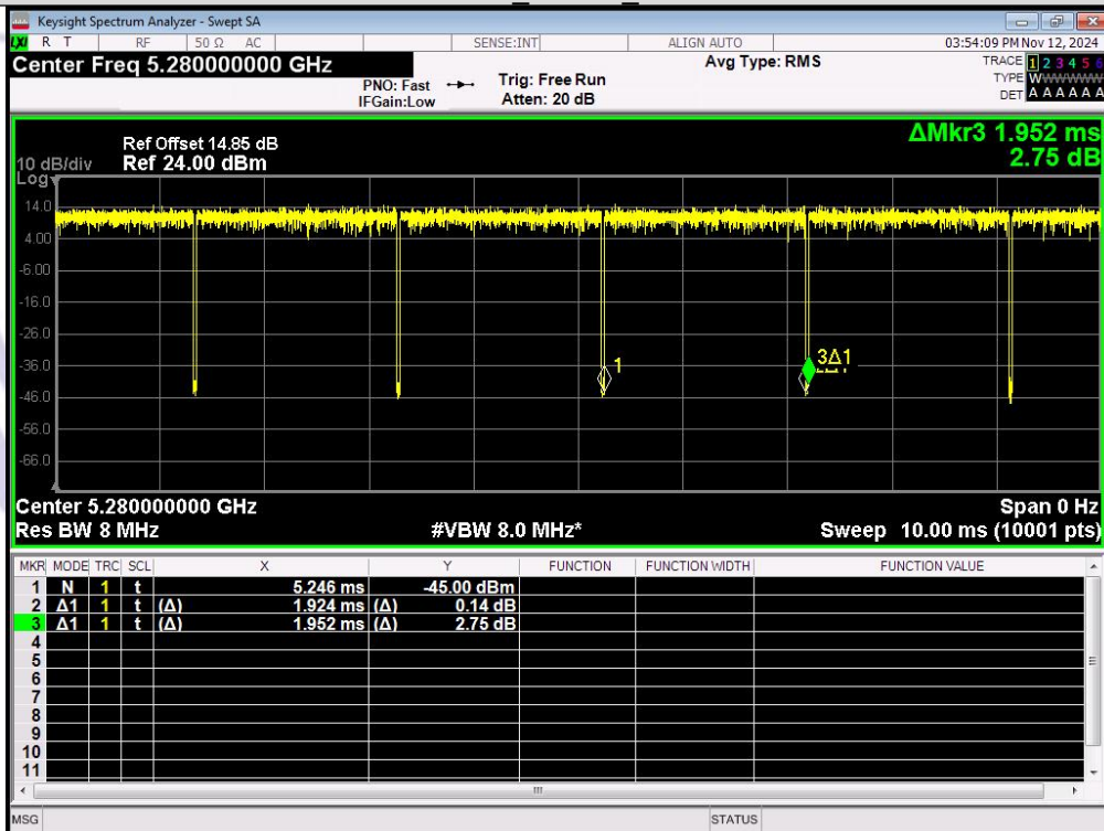
IEEE 802.11n_20MHz_Channel 56
