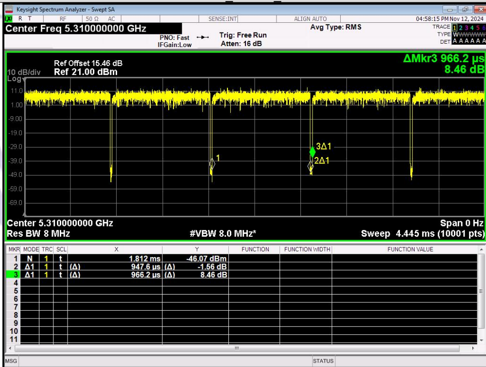
IEEE 802.11n_40MHz_Channel 62
