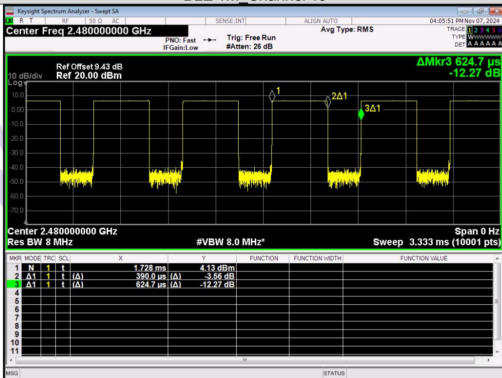
BLE 1M_Channel 39
