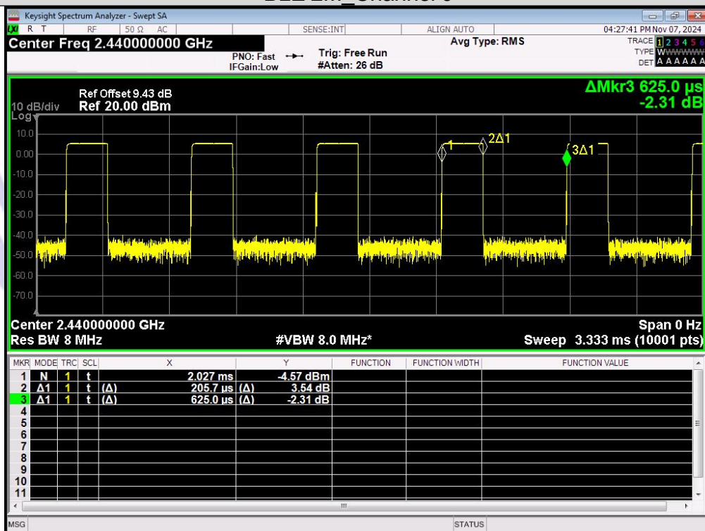
BLE 2M_Channel 19
