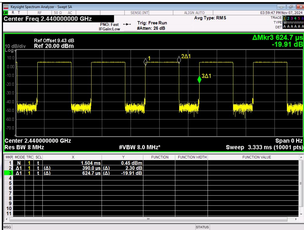
BLE 1M_Channel 19
