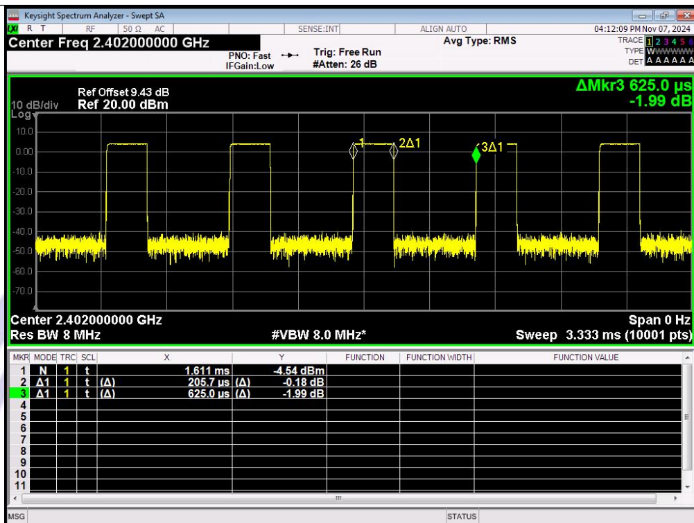
BLE 2M_Channel 0
