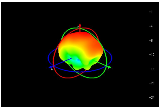
Main: 2400Mhz
