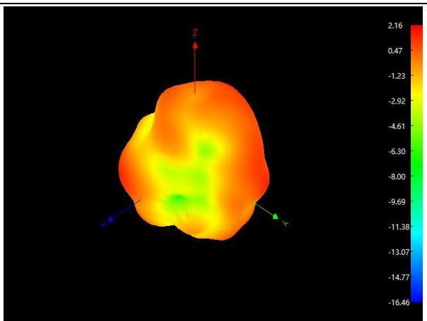
BT/WIFI: 2450Mhz
