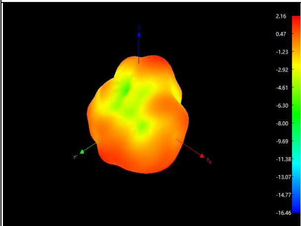
BT/WIFI: 2420Mhz
