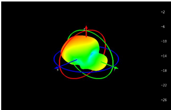
Main: 1700Mhz
