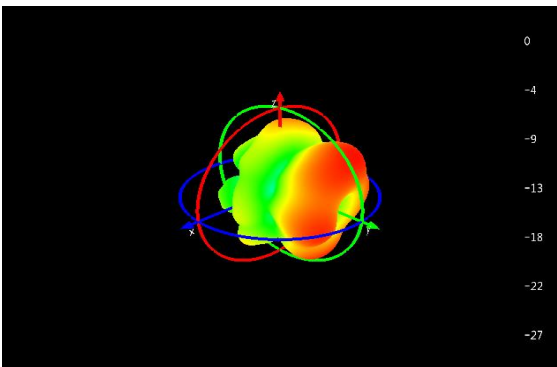
Main: 2100Mhz
