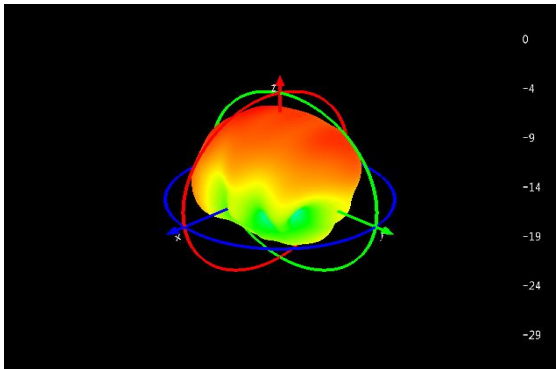
Main: 2600Mhz
