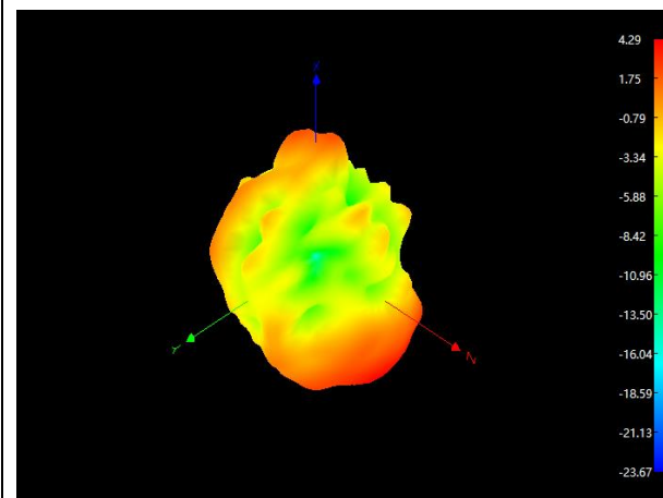
BT/WIFI: 2480Mhz
