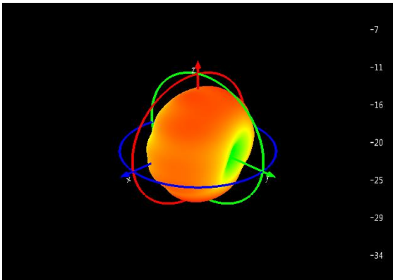
Main: 800Mhz
