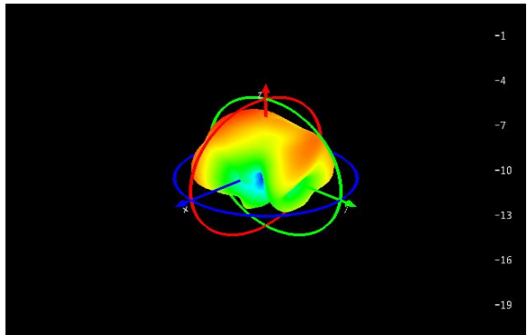
Main: 1900Mhz
