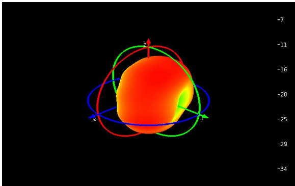
Main: 900Mhz
