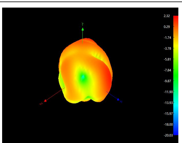
Main: 900Mhz
