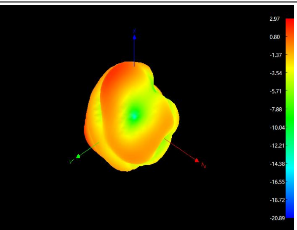
Main: 1900Mhz
