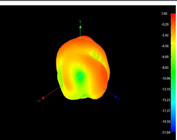
Main: 700Mhz
