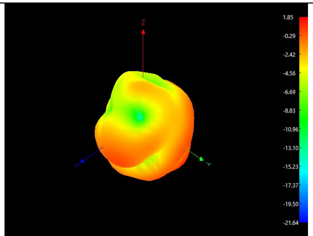
Main: 800Mhz
