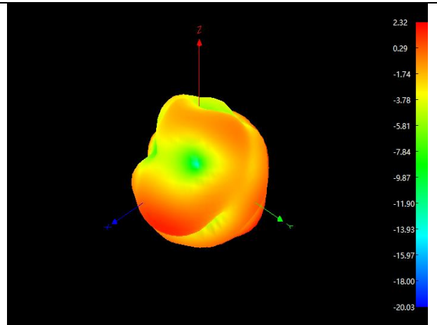
Main: 1700Mhz
