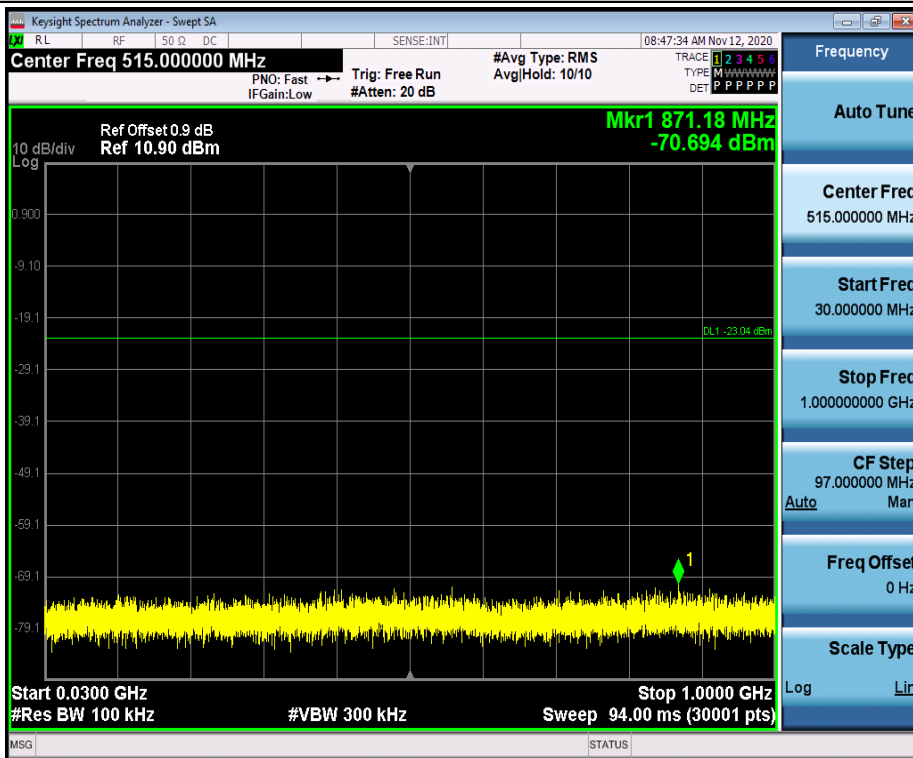
11B_Ant1_2462_30~1000
