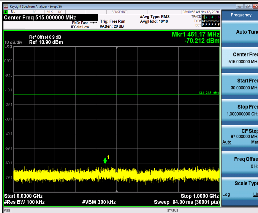
11B_Ant1_2412_30~1000
