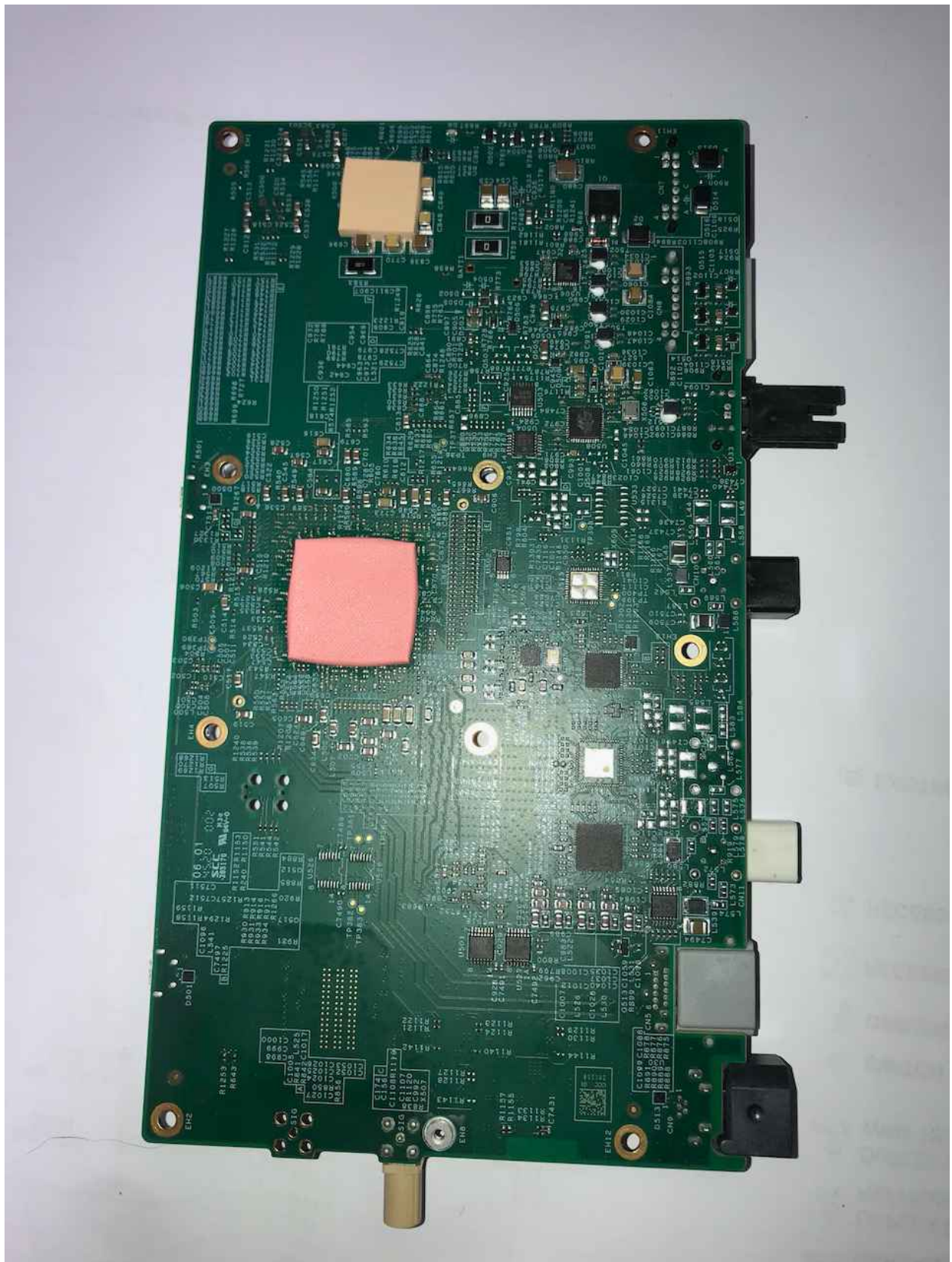
PCB Bottom
