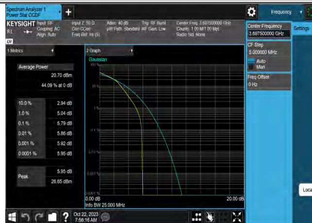
Band48-10MHz-QPSK-55290-1RB#0
