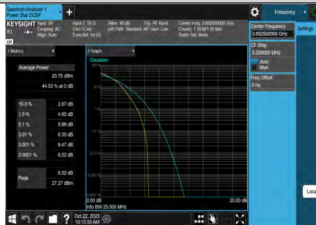
Band48-20MHz-QPSK-55340-1RB#0
