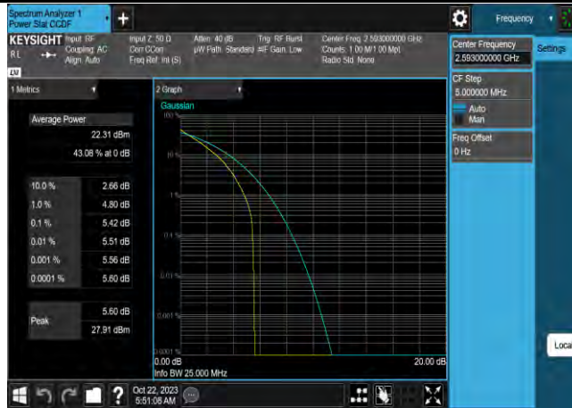
Band41-5MHz-QPSK-41565-1RB#0
