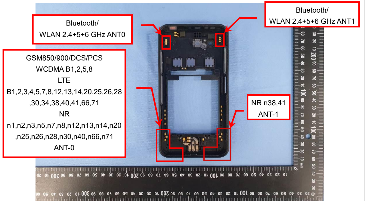
EUT Photo (2)
