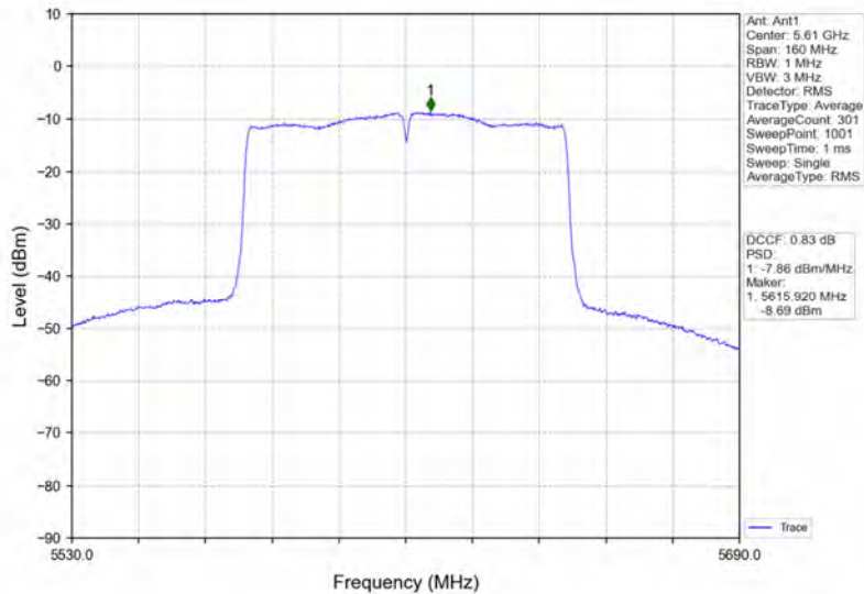
802.11ac(VHT80)_HCH_5610MHz_Ant1_NTNV
