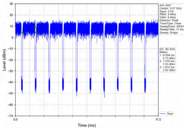
802.11ac(VHT40)_LCH_5270MHz_Ant1_NTNV
