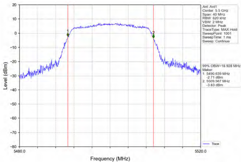
802.11ac(VHT20)_LCH_5500MHz_Ant1_NTNV
