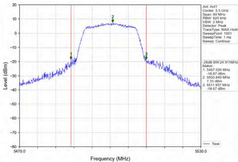
802.11n(HT20)_LCH_5500MHz_Ant1_NTNV
