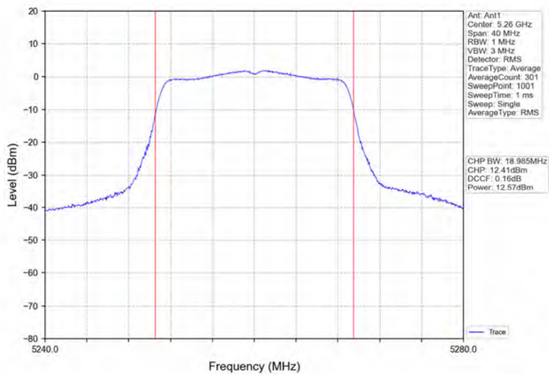
802.11n(HT20)_LCH_5260MHz_Ant1_NTNV
