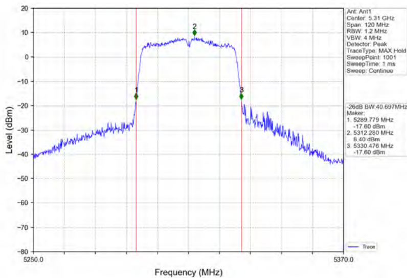
802.11n(HT40)_HCH_5310MHz_Ant1_NTNV
