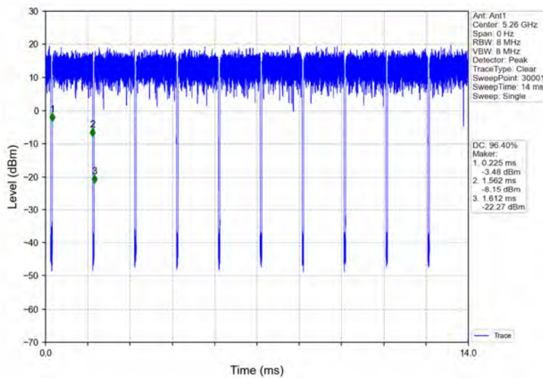
802.11n(HT20)_LCH_5260MHz_Ant1_NTNV
