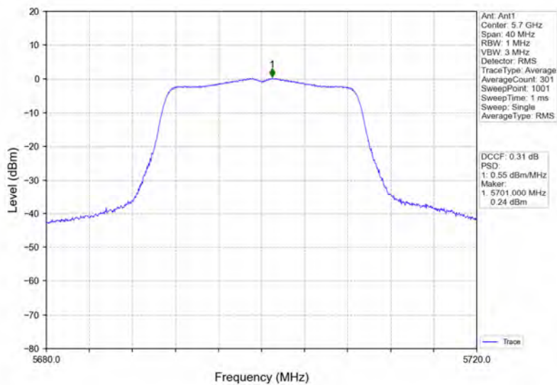
802.11ac(VHT20)_HCH_5700MHz_Ant1_NTNV
