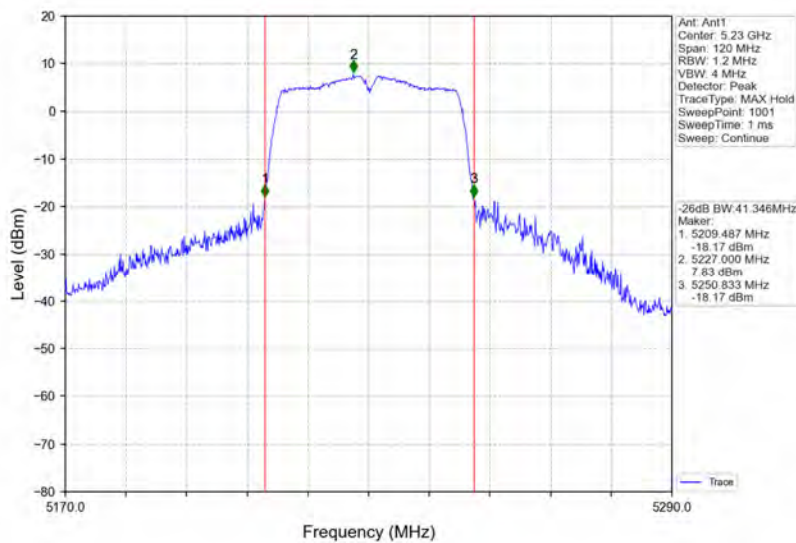
802.11ac(VHT40)_HCH_5230MHz_Ant1_NTNV
