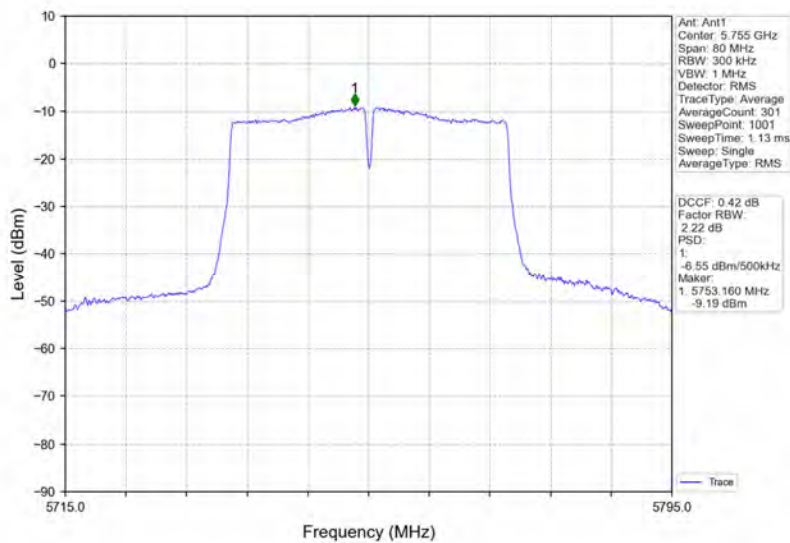
802.11ac(VHT40)_LCH_5755MHz_Ant1_NTNV
