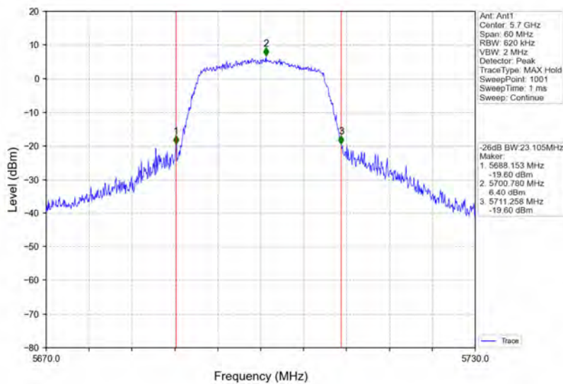
802.11ac(VHT20)_HCH_5700MHz_Ant1_NTNV
