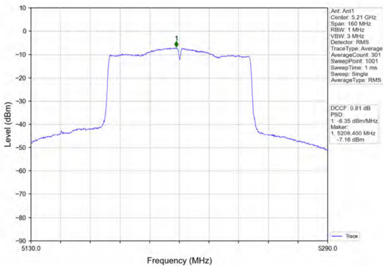
802.11ac(VHT80)_MCH_5210MHz_Ant1_NTNV
