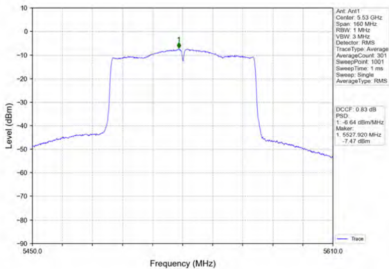
802.11ac(VHT80)_LCH_5530MHz_Ant1_NTNV
