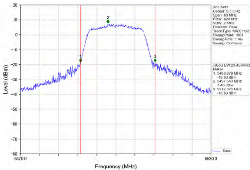
802.11ac(VHT20)_LCH_5500MHz_Ant1_NTNV
