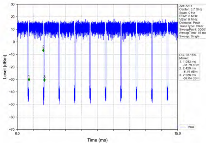
802.11ac(VHT20)_HCH_5700MHz_Ant1_NTNV
