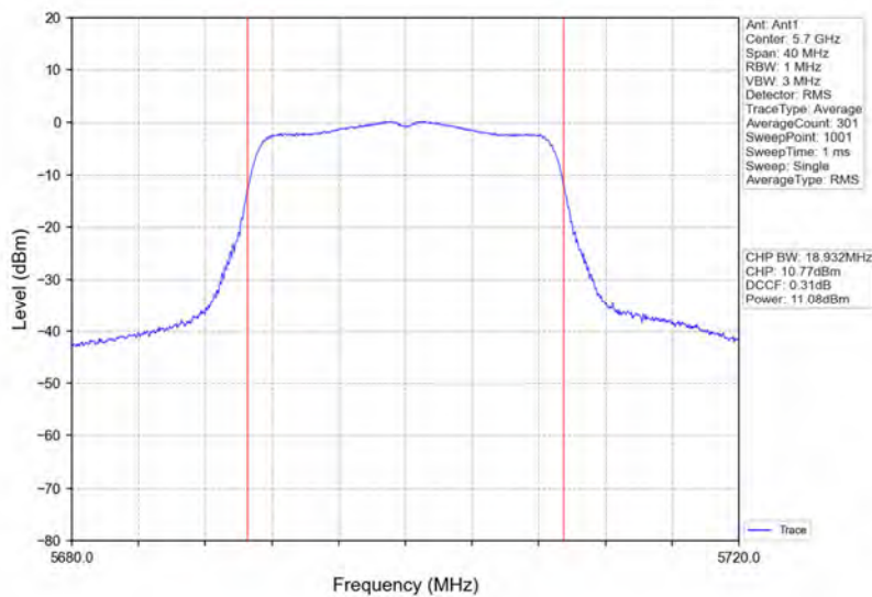
802.11ac(VHT20)_HCH_5700MHz_Ant1_NTNV
