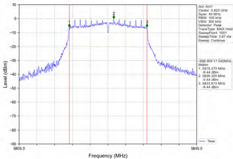
802.11n(HT20)_HCH_5825MHz_Ant1_NTNV
