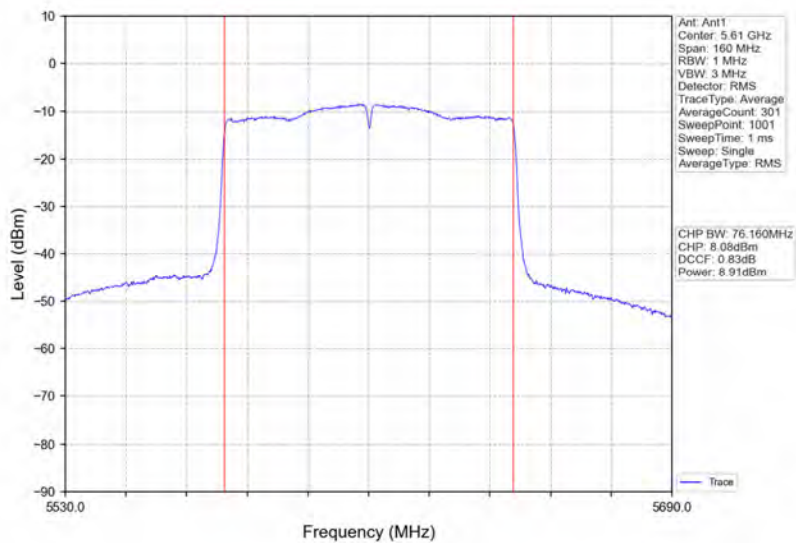
802.11ac(VHT80)_HCH_5610MHz_Ant1_NTNV
