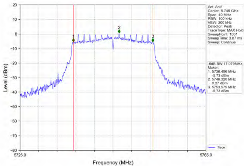
802.11n(HT20)_LCH_5745MHz_Ant1_NTNV
