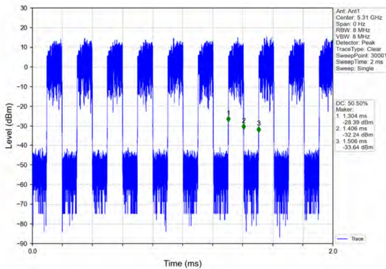
802.11n(HT40)_HCH_5310MHz_Ant1_NTNV
