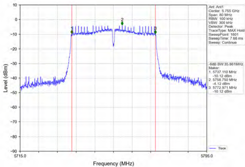
802.11ac(VHT40)_LCH_5755MHz_Ant1_NTNV
