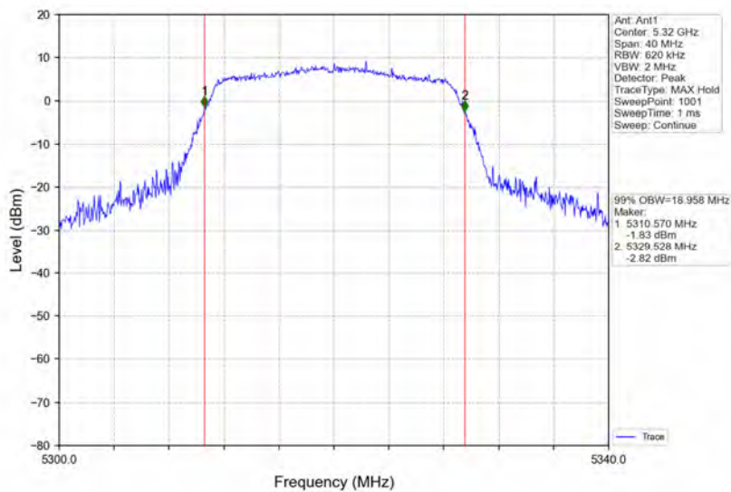
802.11n(HT20)_HCH_5320MHz_Ant1_NTNV
