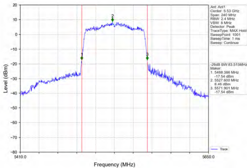
802.11ac(VHT80)_LCH_5530MHz_Ant1_NTNV
