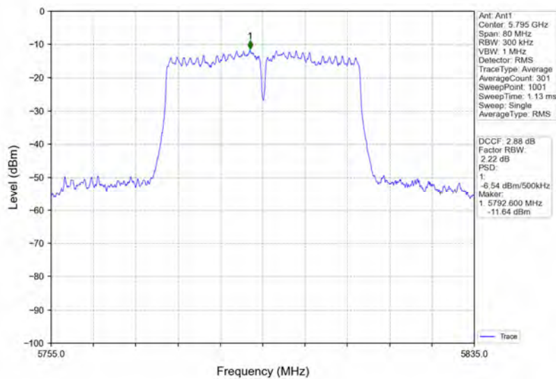
802.11n(HT40)_HCH_5795MHz_Ant1_NTNV
