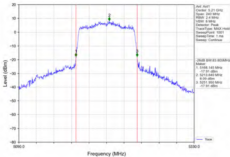
802.11ac(VHT80)_MCH_5210MHz_Ant1_NTNV
