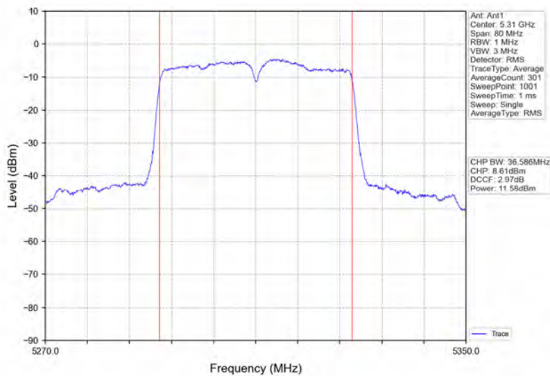
802.11n(HT40)_HCH_5310MHz_Ant1_NTNV
