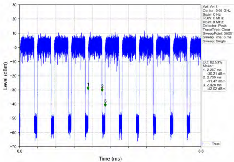
802.11ac(VHT80)_HCH_5610MHz_Ant1_NTNV
