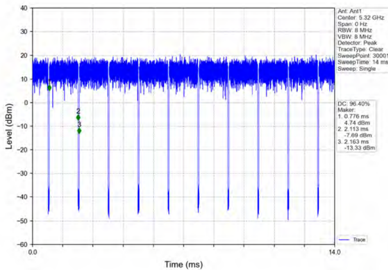
802.11n(HT20)_HCH_5320MHz_Ant1_NTNV
