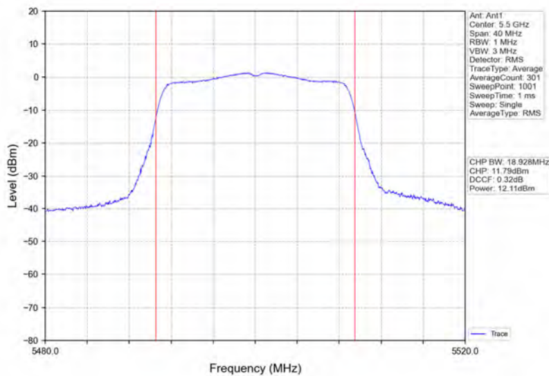
802.11ac(VHT20)_LCH_5500MHz_Ant1_NTNV
