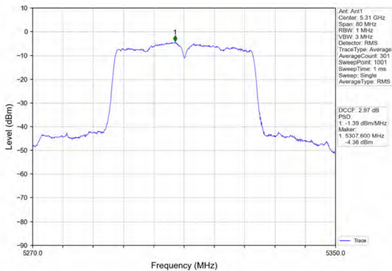
802.11n(HT40)_HCH_5310MHz_Ant1_NTNV
