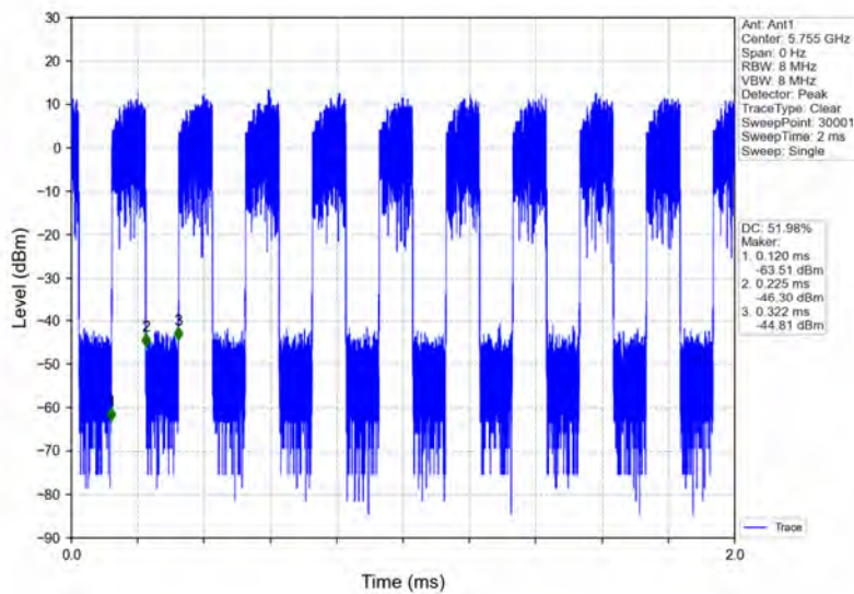
802.11n(HT40)_LCH_5755MHz_Ant1_NTNV
