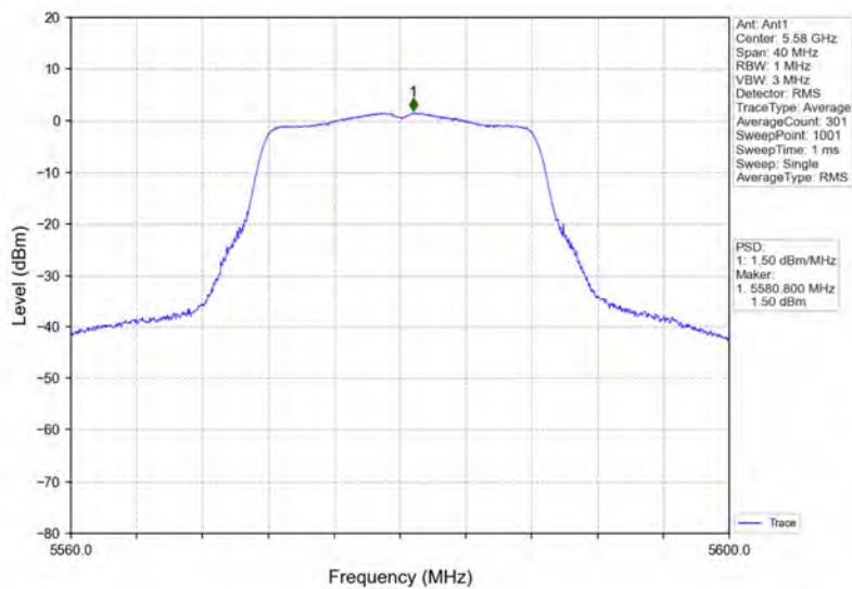
802.11a_MCH_5580MHz_Ant1_NTNV
