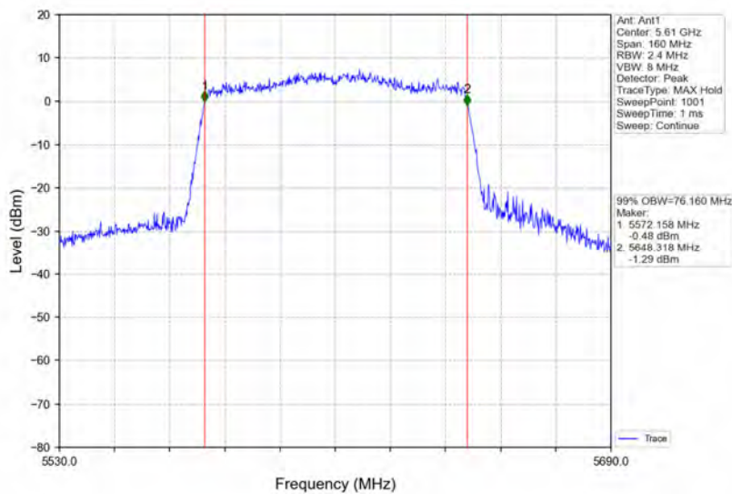
802.11ac(VHT80)_HCH_5610MHz_Ant1_NTNV
