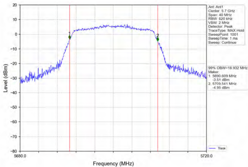
802.11ac(VHT20)_HCH_5700MHz_Ant1_NTNV
