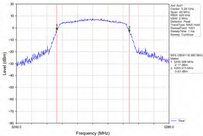
802.11n(HT20)_LCH_5260MHz_Ant1_NTNV
