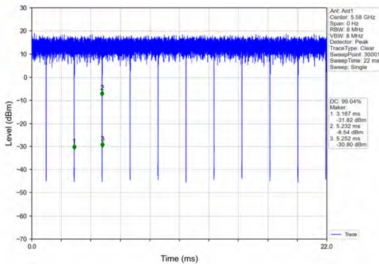
802.11a_MCH_5580MHz_Ant1_NTNV
