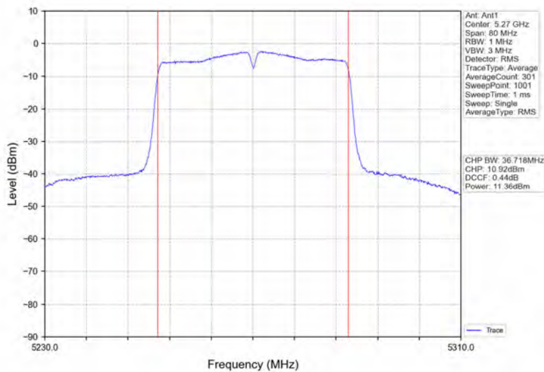
802.11ac(VHT40)_LCH_5270MHz_Ant1_NTNV
