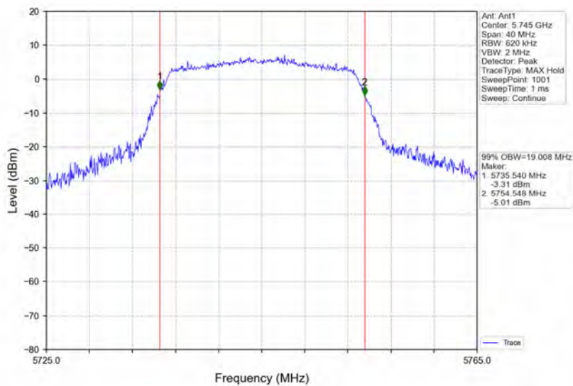
802.11n(HT20)_LCH_5745MHz_Ant1_NTNV
