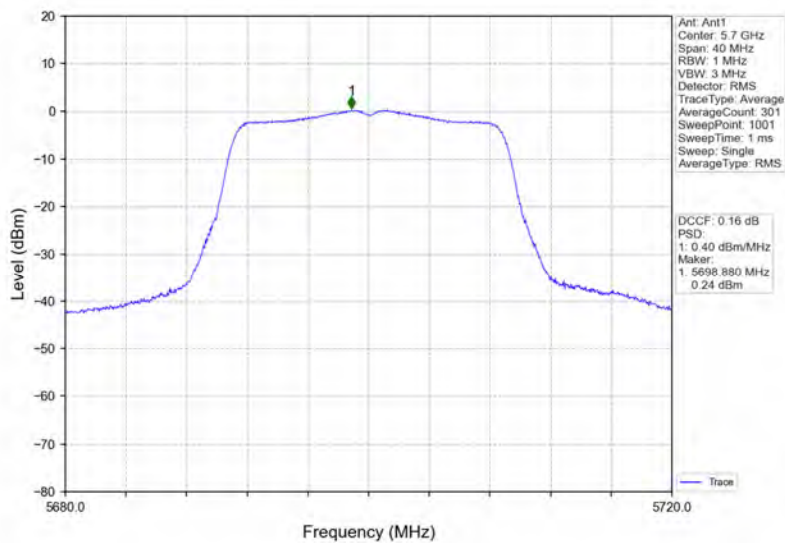
802.11n(HT20)_HCH_5700MHz_Ant1_NTNV
