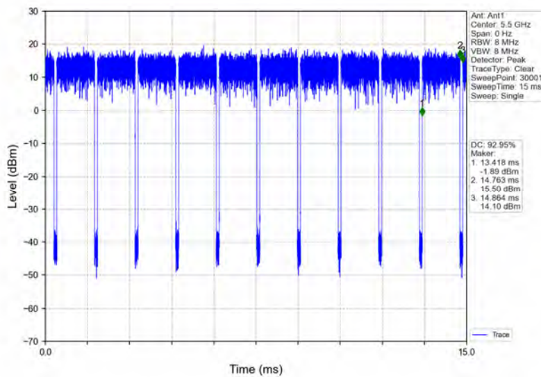
802.11ac(VHT20)_LCH_5500MHz_Ant1_NTNV
