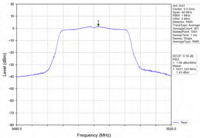
802.11n(HT20)_LCH_5500MHz_Ant1_NTNV
