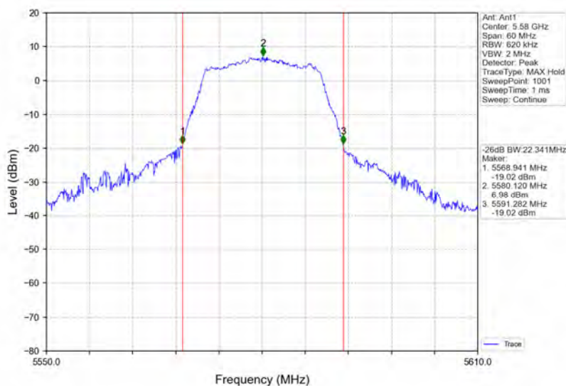
802.11a_MCH_5580MHz_Ant1_NTNV
