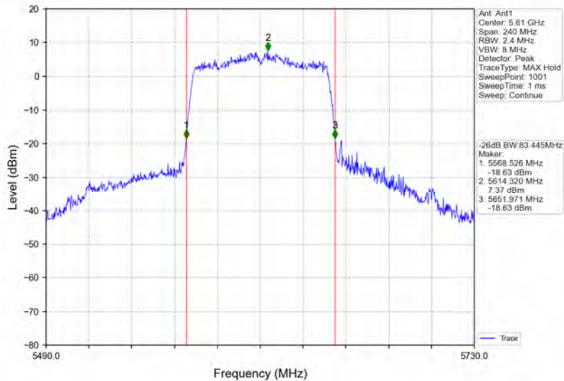
802.11ac(VHT80)_HCH_5610MHz_Ant1_NTNV
