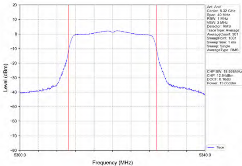
802.11n(HT20)_HCH_5320MHz_Ant1_NTNV
