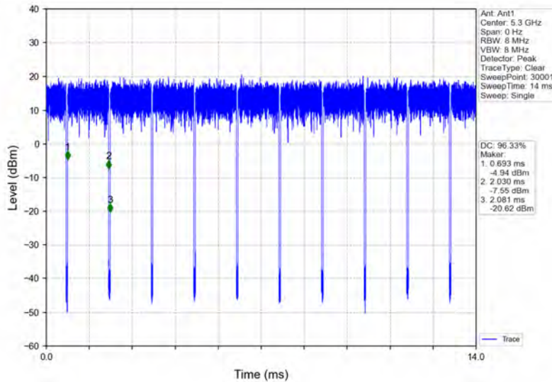
802.11n(HT20)_HCH_5320MHz_Ant1_NTNV
