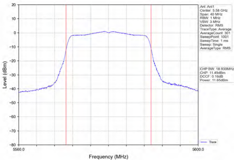
802.11n(HT20)_MCH_5580MHz_Ant1_NTNV
