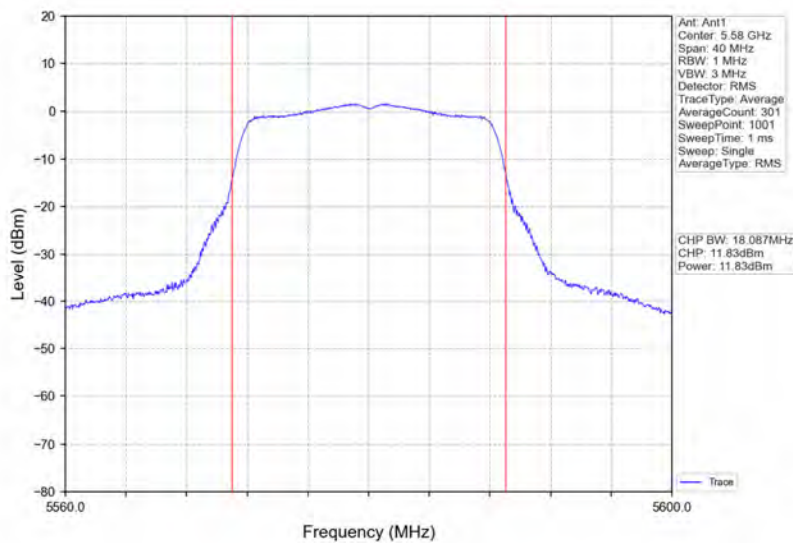
802.11a_MCH_5580MHz_Ant1_NTNV
