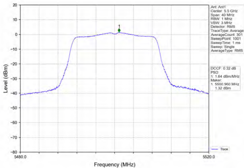
802.11ac(VHT20)_LCH_5500MHz_Ant1_NTNV
