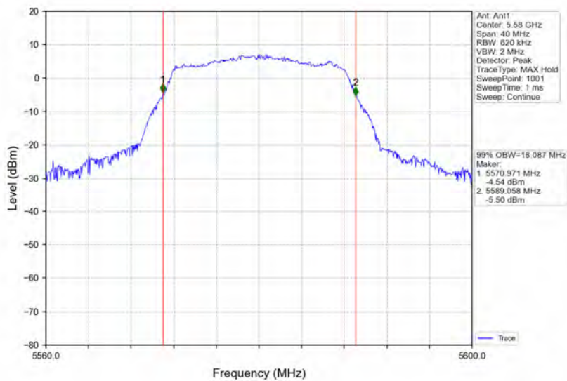
802.11a_MCH_5580MHz_Ant1_NTNV
