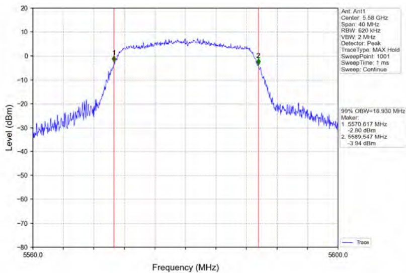
802.11n(HT20)_MCH_5580MHz_Ant1_NTNV
