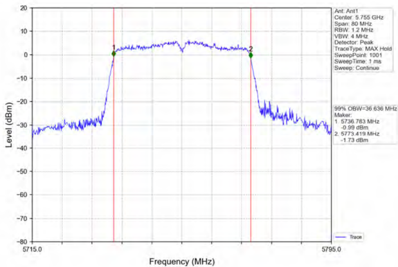
802.11n(HT40)_LCH_5755MHz_Ant1_NTNV
