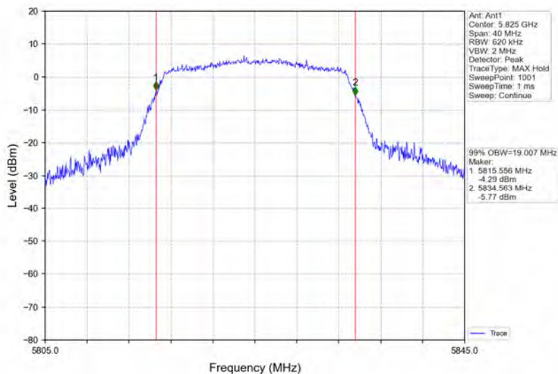
802.11n(HT20)_HCH_5825MHz_Ant1_NTNV
