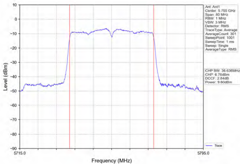
802.11n(HT40)_LCH_5755MHz_Ant1_NTNV
