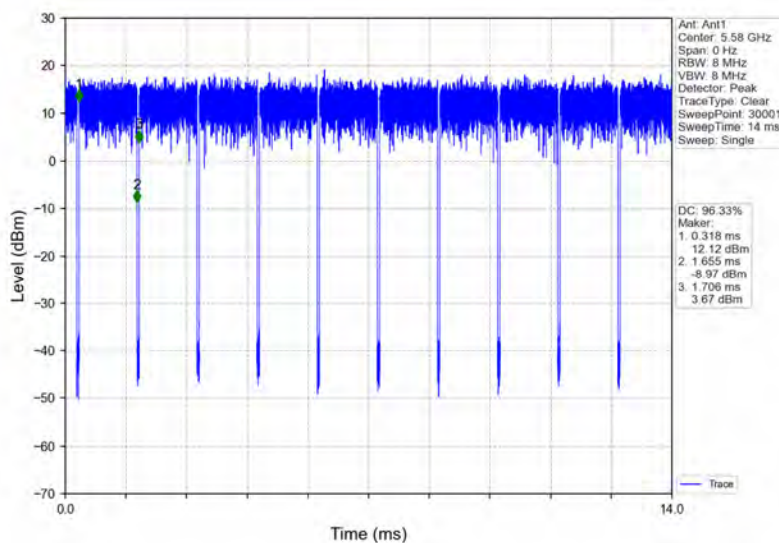
802.11n(HT20)_MCH_5580MHz_Ant1_NTNV
