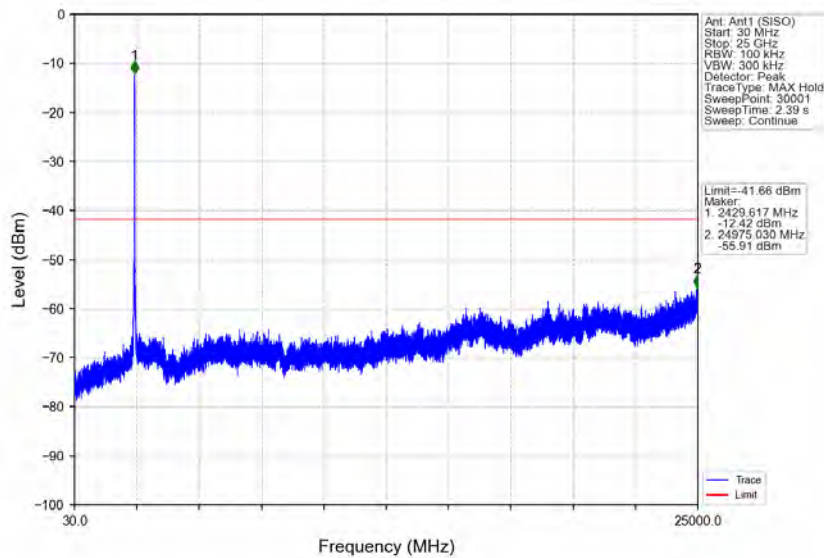
802.11n(HT40)_MCH_2437MHz_Ant1 (SISO)_NTNV
