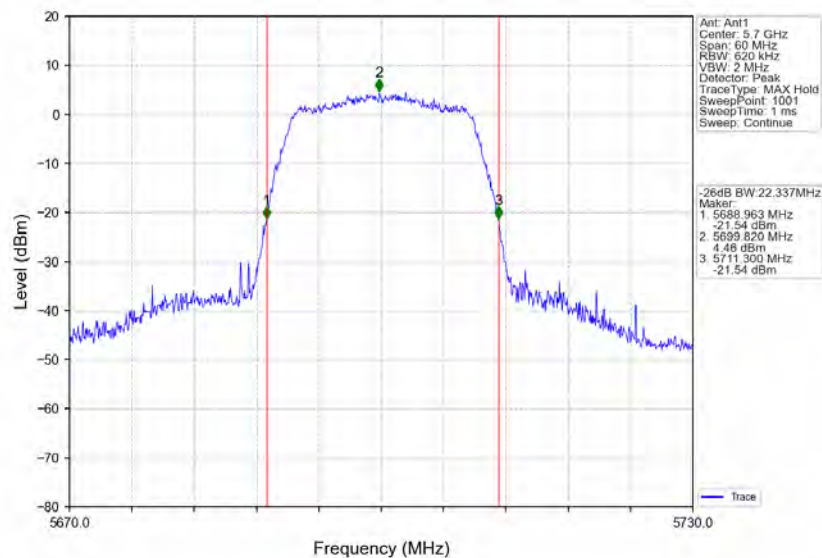
802.11ac(VHT20)_HCH_5700MHz_Ant1_NTNV
