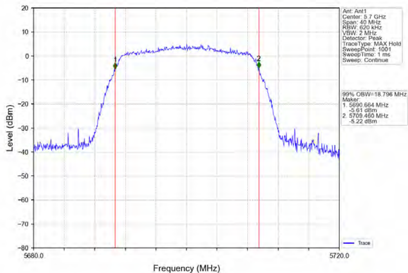
802.11ac(VHT20)_HCH_5700MHz_Ant1_NTNV
