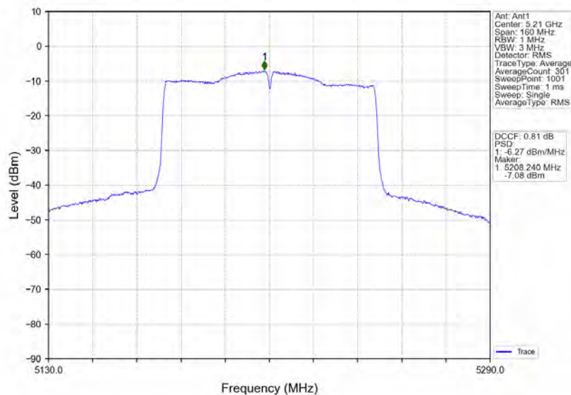
802.11ac(VHT80)_MCH_5210MHz_Ant1_NTNV
