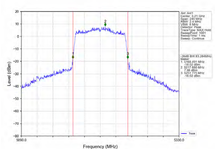
802.11ac(VHT80)_MCH_5210MHz_Ant1_NTNV
