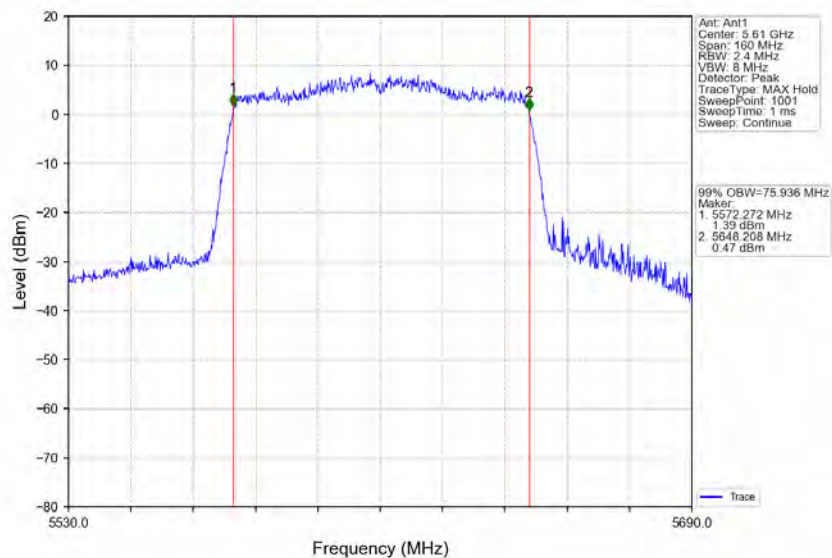
802.11ac(VHT80)_HCH_5610MHz_Ant1_NTNV
