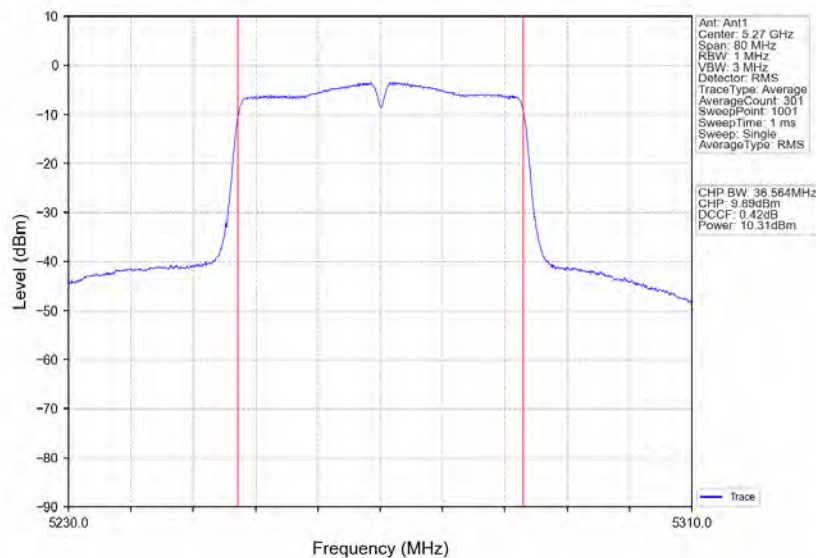
802.11ac(VHT40)_LCH_5270MHz_Ant1_NTNV
