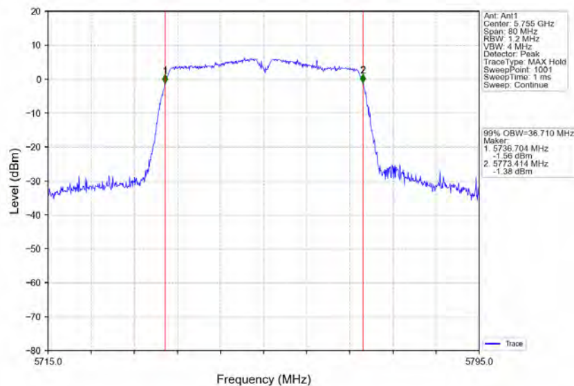
802.11n(HT40)_LCH_5755MHz_Ant1_NTNV
