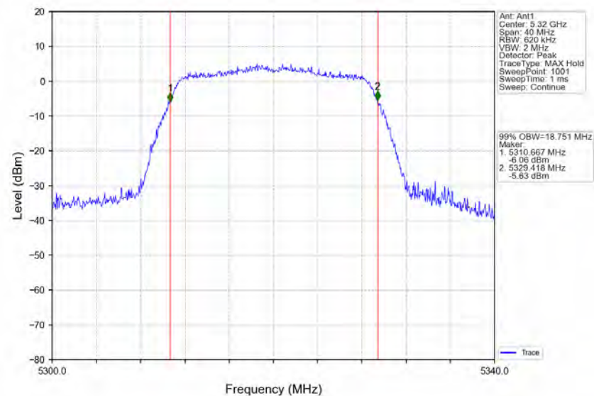
802.11n(HT20)_HCH_5320MHz_Ant1_NTNV
