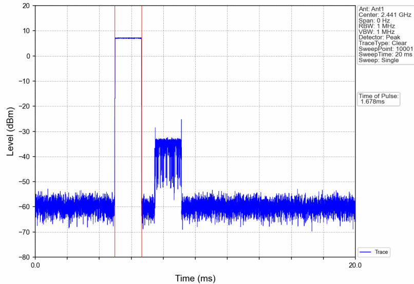
GFSK_DH3_HOPP_Ant1_NTNV
