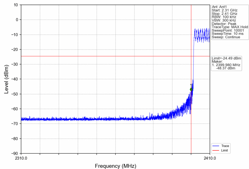
8DPSK_3DH5_HOPP_Ant1_NTNV
