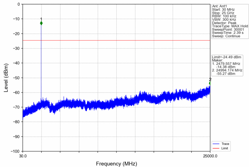
8DPSK_3DH5_HOPP_Ant1_NTNV
