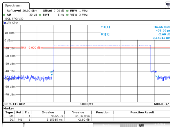
DH5_Hopping 3.153ms
