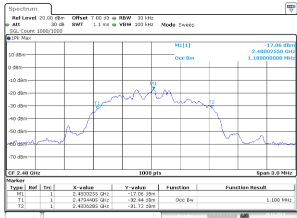
2DH1_High 1.188MHz
