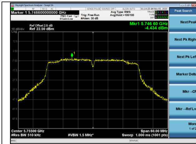
802.11n(HT40) 5755
