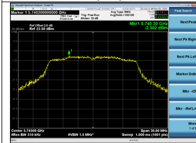
802.11ac(HT20) 5745
