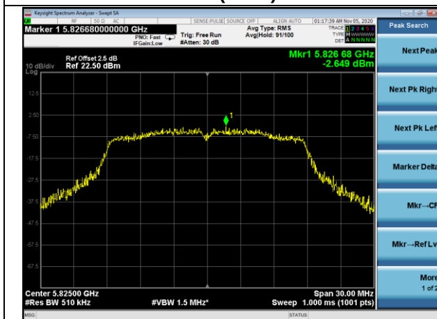
802.11ac(HT20) 5825
