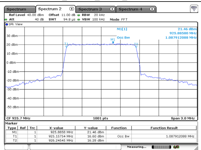
Cat-M1_1.4MHz_QPSK_925.7 MHz
