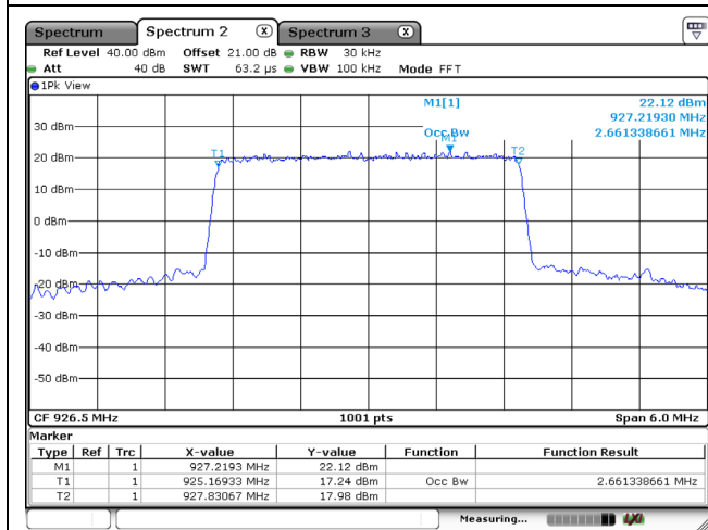
Cat-1_3MHz_QPSK_926.5 MHz
