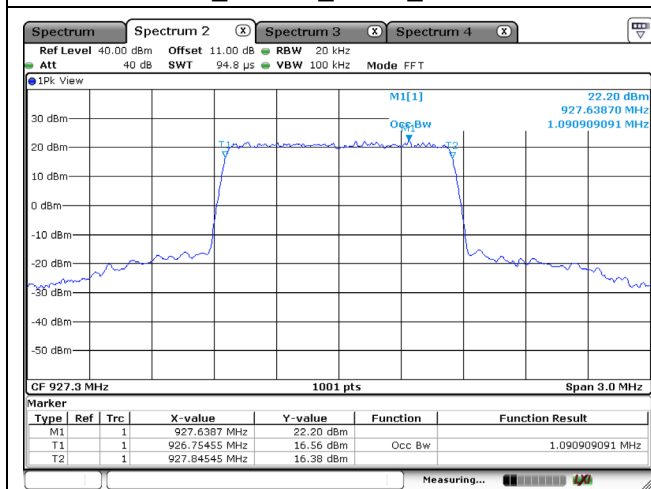
Cat-M1_1.4MHz_QPSK_927.3 MHz
