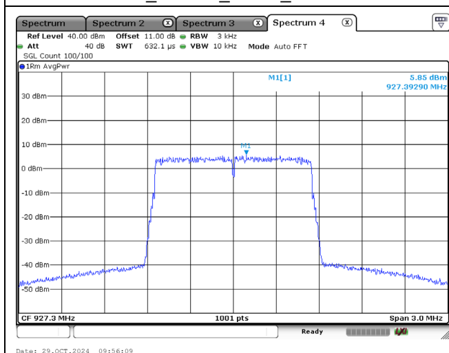
Cat-M1_1.4MHz_QPSK_927.3 MHz
