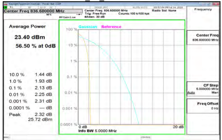
WCDMA B5 MidCH4183-836.6
