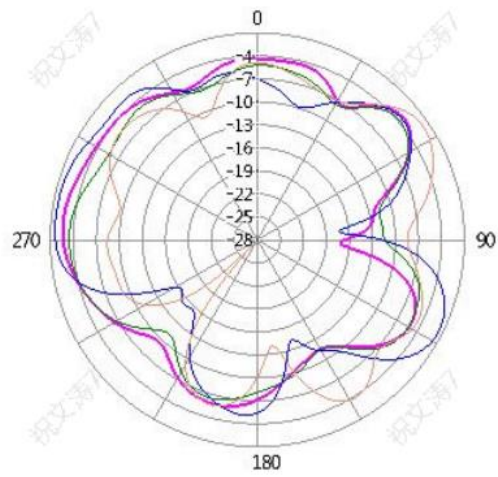
Theta=90 deg
