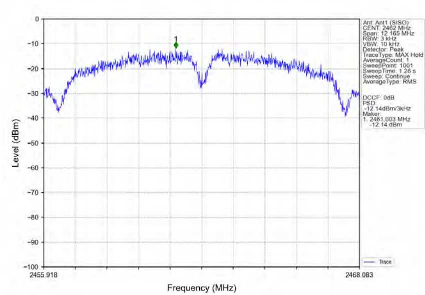
802.11b HCH 2462MHz Ant1 (SISO) NTNV
