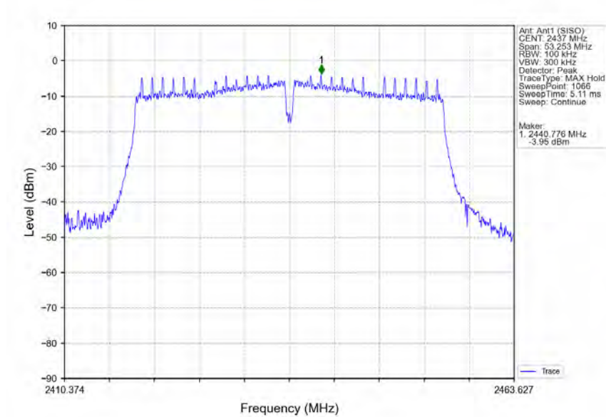
802.11n(HT40) MCH 2437MHz Ant1 (SISO) NTN
