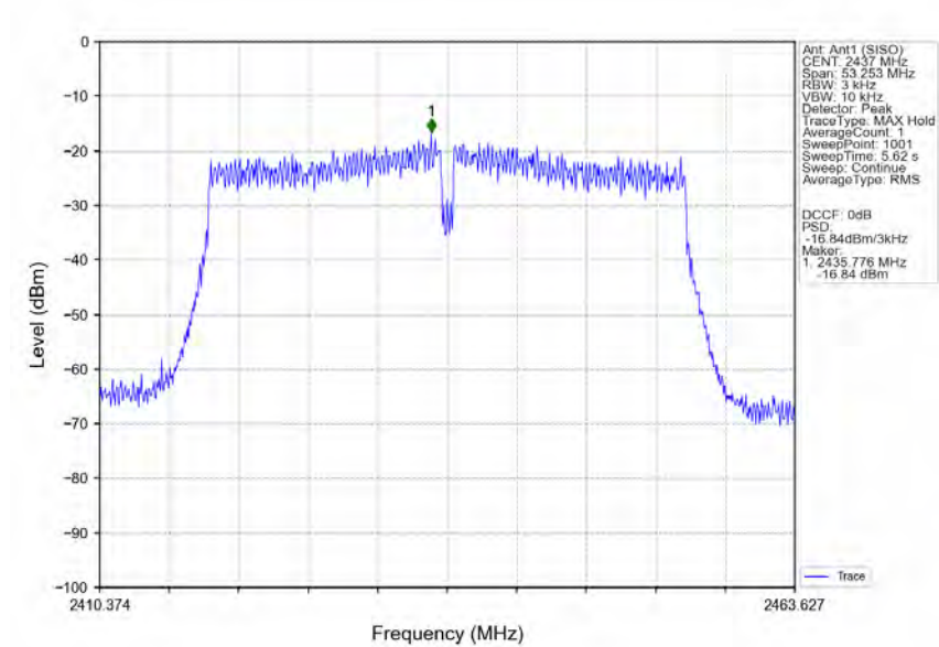
802.11n(HT40) MCH 2437MHz Ant1 (SISO) NTNV
