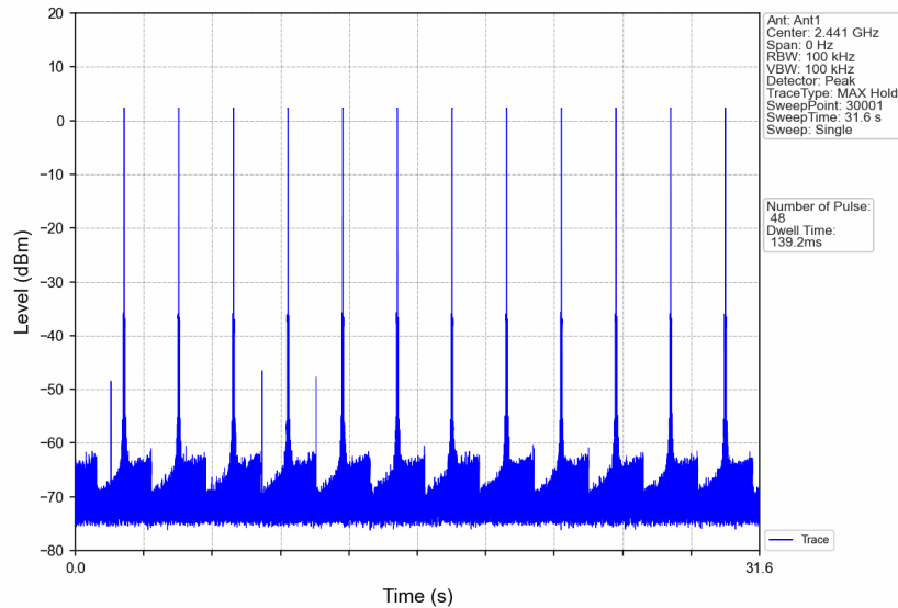
Pi/4DQPSK_2DH1_HOPP_Ant1_NTNV
