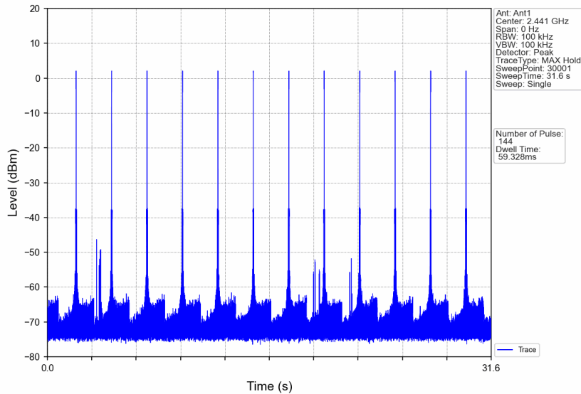
Pi/4DQPSK_2DH3_HOPP_Ant1_NTNV
