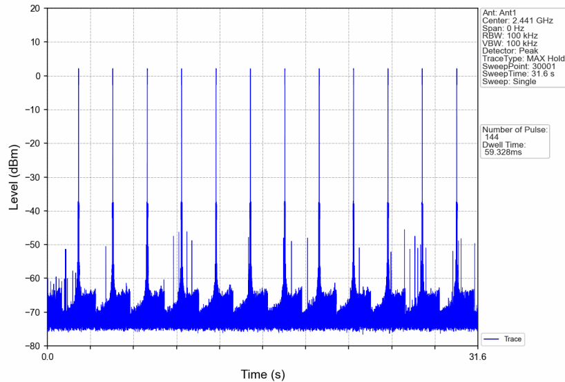
8DPSK_3DH3_HOPP_Ant1_NTNV
