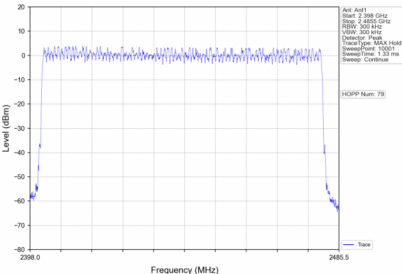
8DPSK_3DH5_HOPP_Ant1_NTNV
