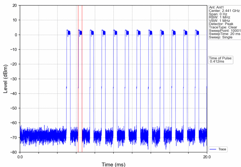
8DPSK_3DH1_HOPP_Ant1_NTNV
