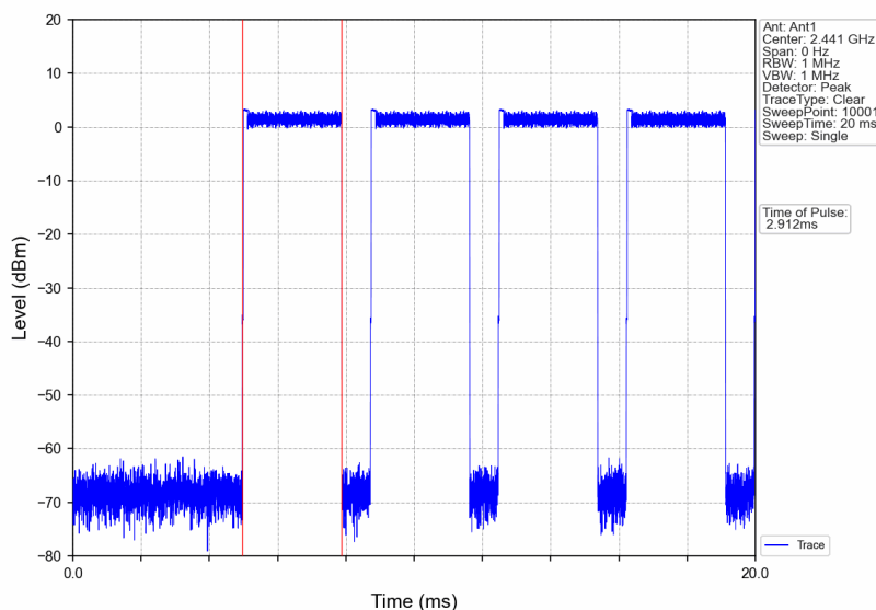
8DPSK_3DH5_HOPP_Ant1_NTNV
