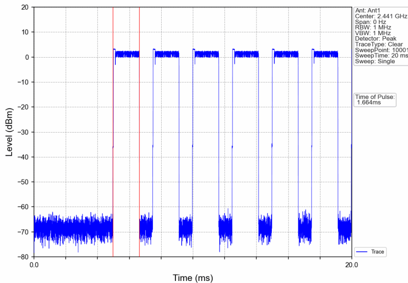
Pi/4DQPSK_2DH3_HOPP_Ant1_NTNV
