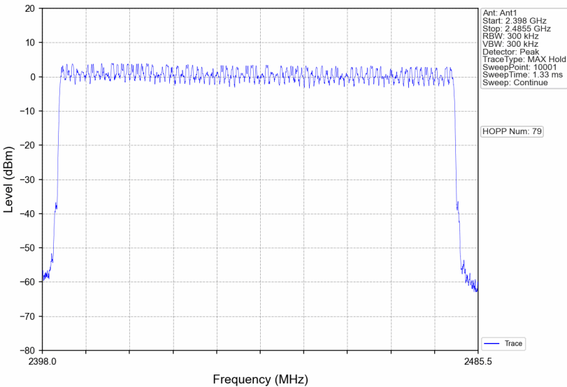
8DPSK_3DH5_HOPP_Ant1_NTNV
