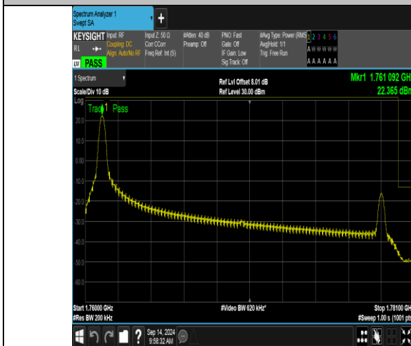
Band66_20MHz_QPSK_132572_1RB#0
