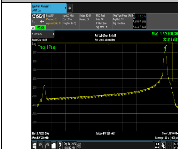
Band66_20MHz_QPSK_132572_1RB#99
