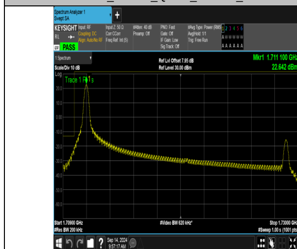
Band66_20MHz_QPSK_132072_1RB#0
