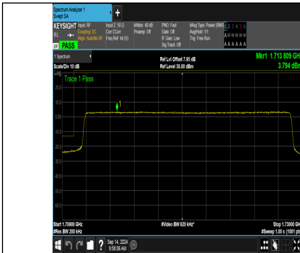
Band66_20MHz_QPSK_132072_100RB#0
