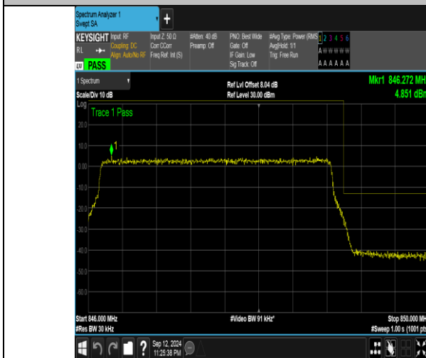
Band5_3MHz_QPSK_20635_15RB#0
