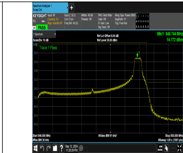
Band5_3MHz_16QAM_20635_1RB#14
