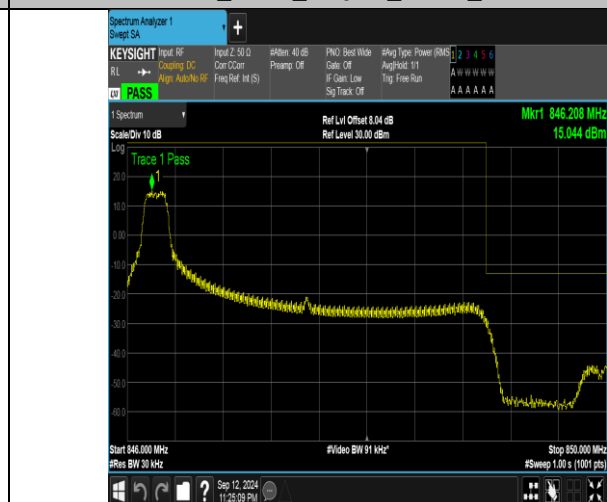
Band5_3MHz_16QAM_20635_1RB#0
