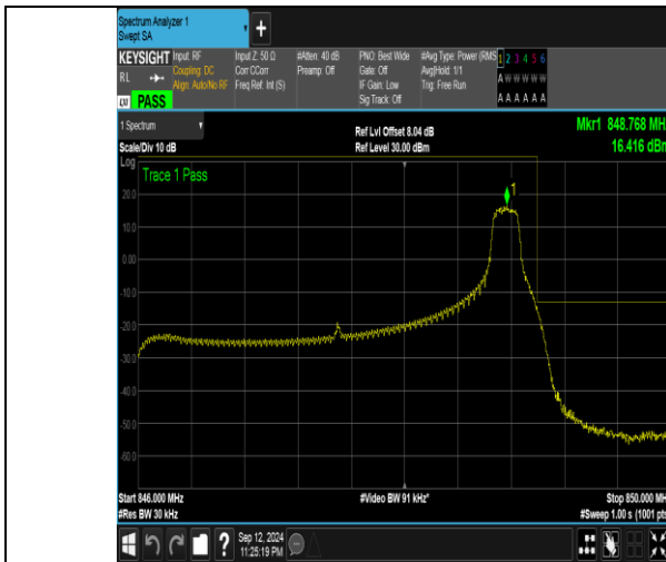
Band5_3MHz_QPSK_20635_1RB#14
