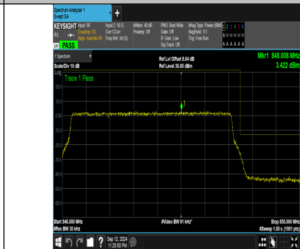
Band5_3MHz_16QAM_20635_15RB#0
