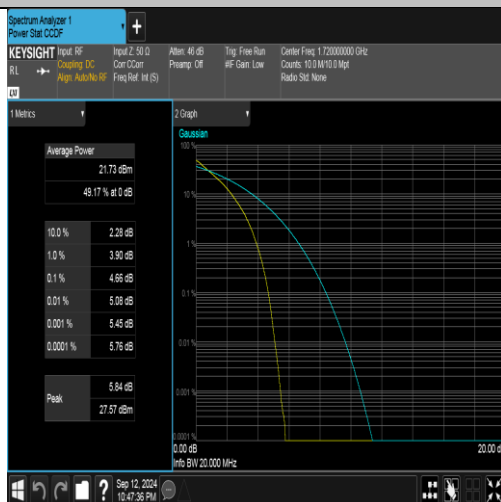
Band4-20MHz-QPSK-20050-100RB#0-PASS
