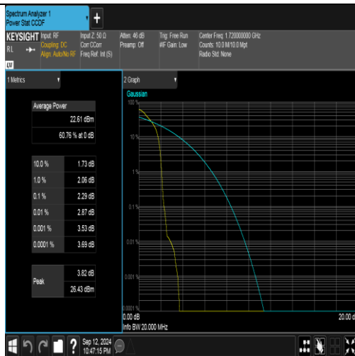
Band4-20MHz-QPSK-20050-1RB#0-PASS
