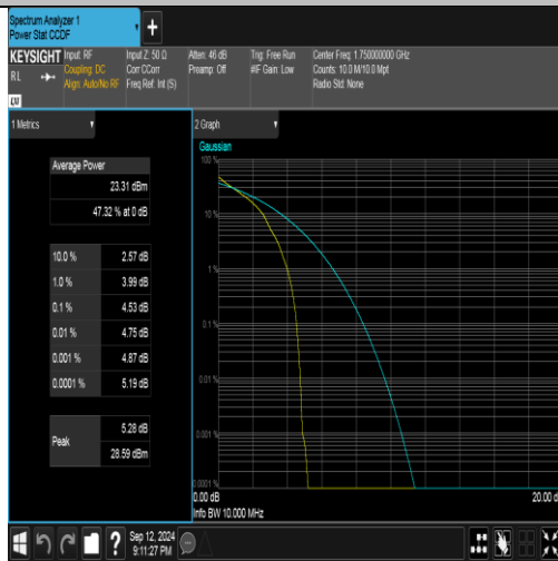
Band4-10MHz-QPSK-20350-1RB#0-PASS
