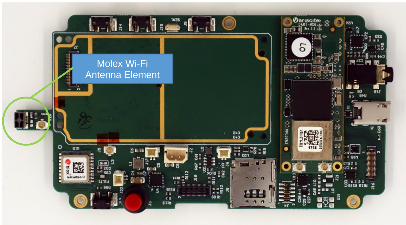
SHOUT sp Main PCBA – Top without 9523 Modem but with the Variscite SoM module
