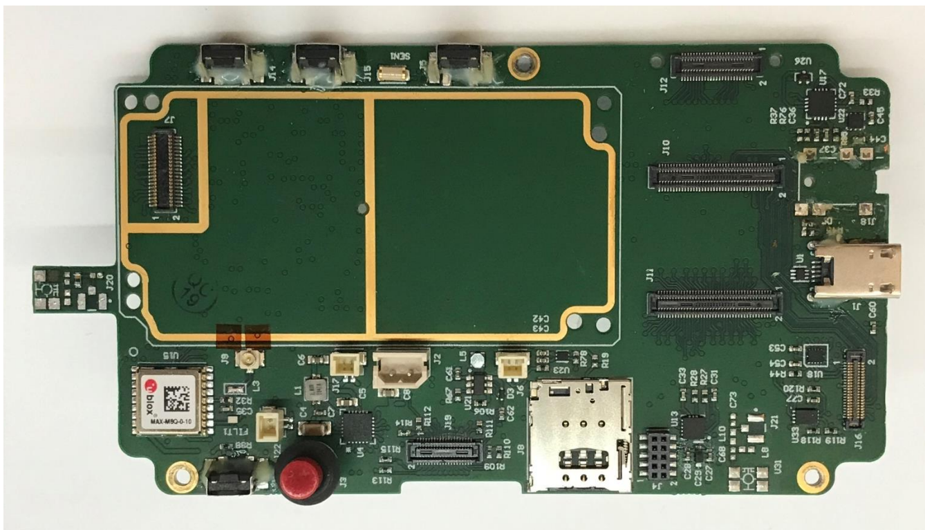
SHOUT sp Main PCBA – Top without 9523 Modem and Variscite SoM module
