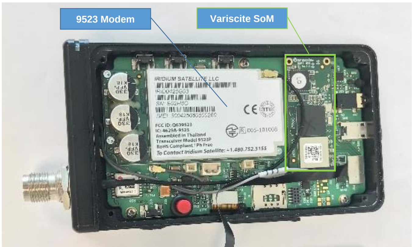
SHOUT sp Main PCBA – Top with 9523 Modem and Variscite SoM module
