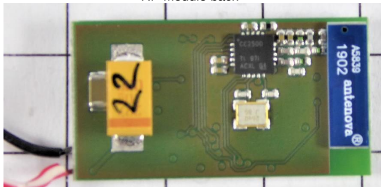
RF-Module back
