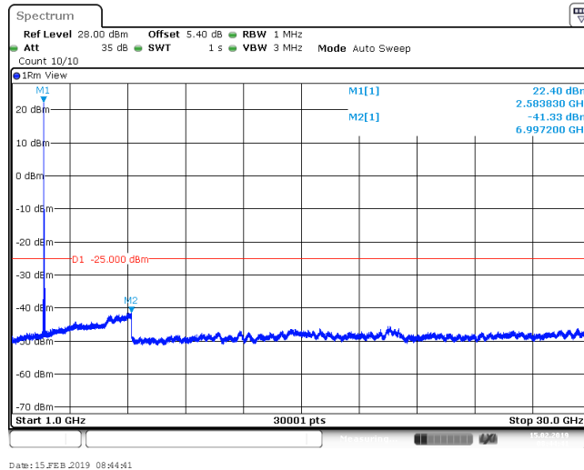
Band41_20MHz_QPSK_41490_1RB#0
