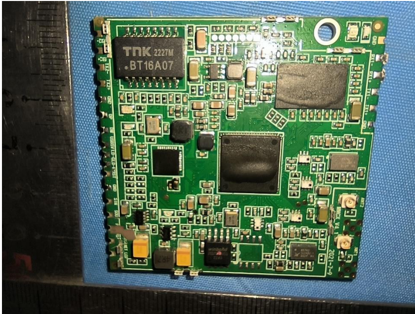
5.8G Module:MK15
