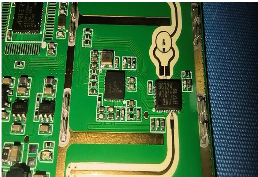
24G Radar Module: TR24DCA100
