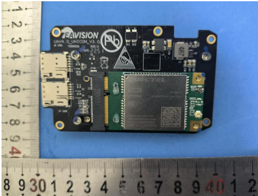
LTE Module: EC20
