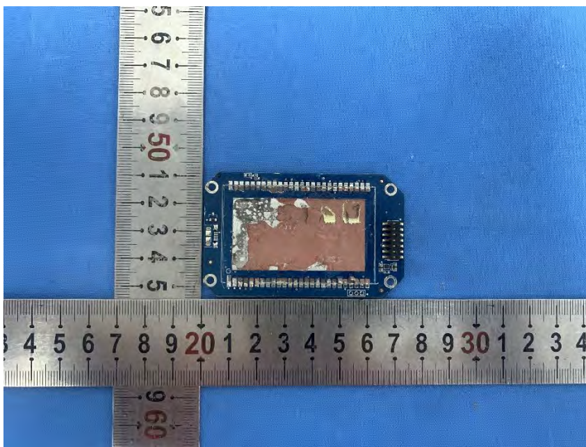
GPS module:OEM7500
