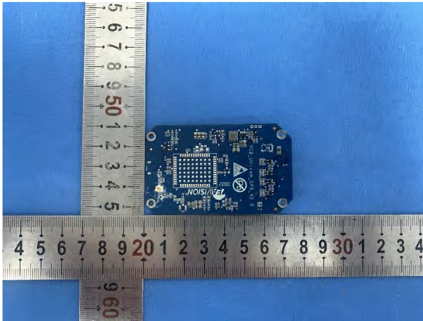
GPS module:OEM7500
