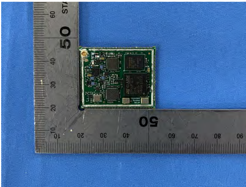
2.4G Proprietary module: P2400
