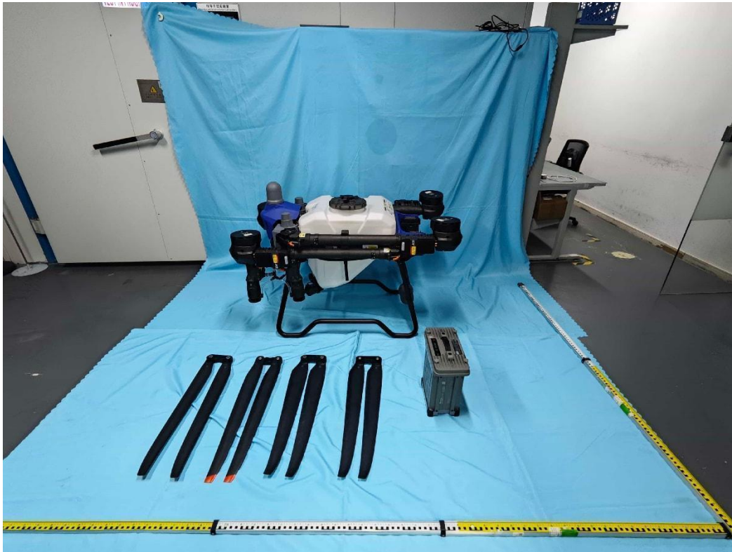
Photo 2 MODEL:EA-J70
