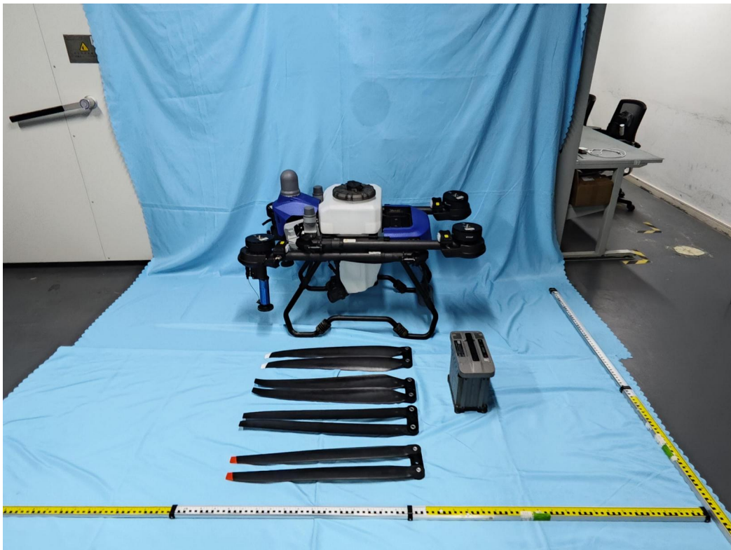
Photo 2 MODEL:EA-J70
