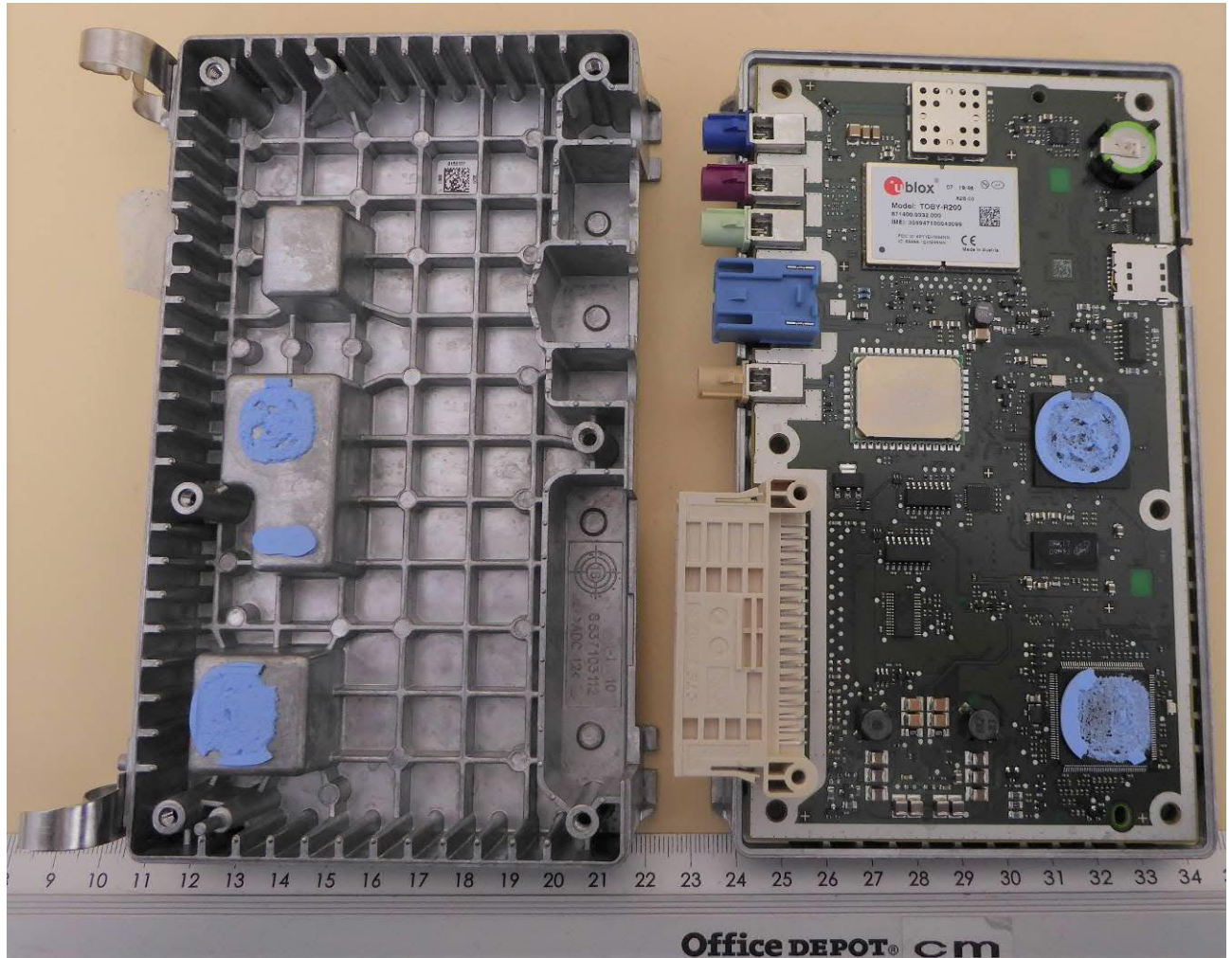
EUT – open 1
