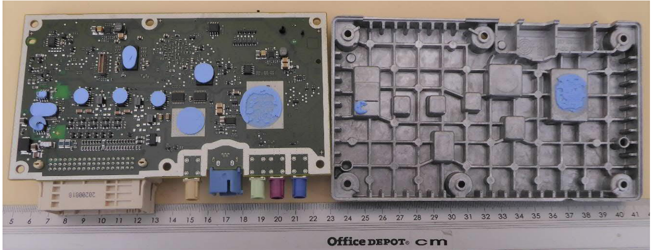
EUT – open 2
