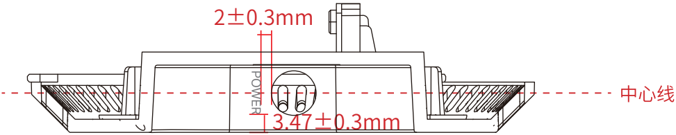
Power接口icon尺寸图
