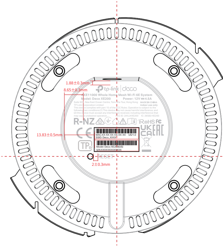
底壳镭雕尺寸图
