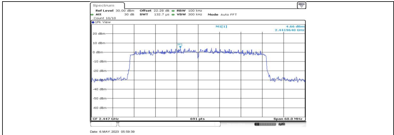
11AX40MIMO_Ant4_2447_0-Reference
