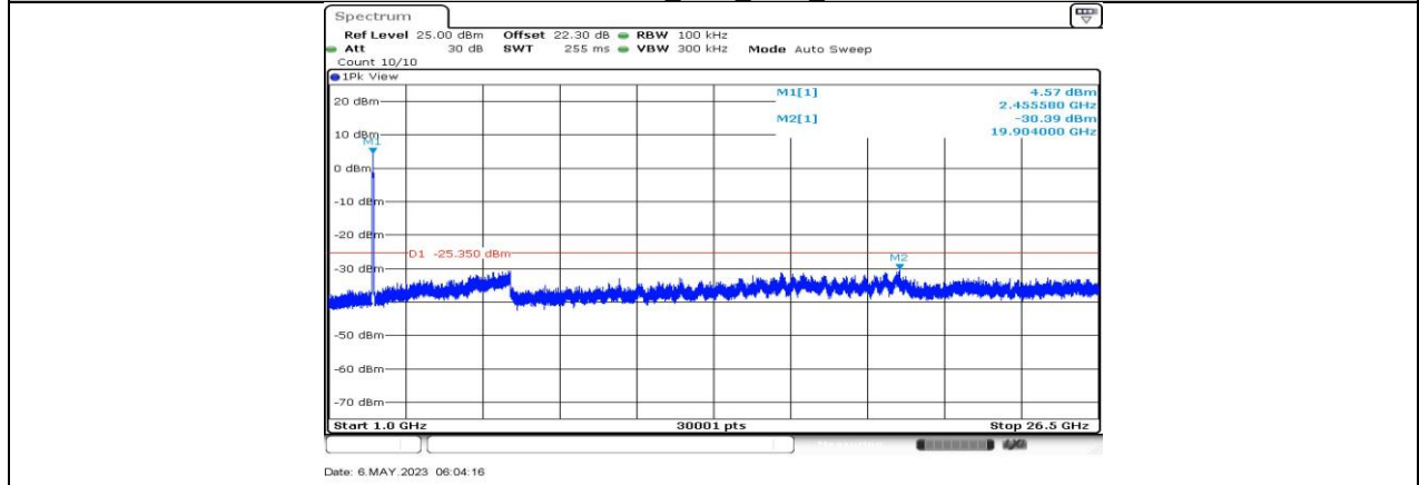
11AX40MIMO_Ant4_2452_1000-26500
