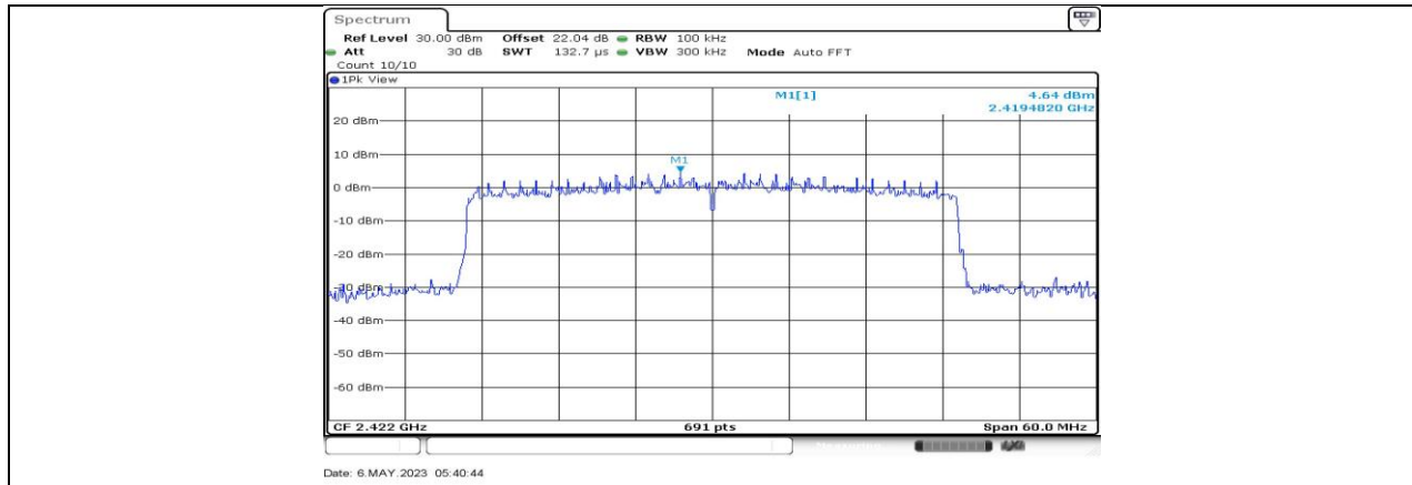
11AX40MIMO_Ant2_2422_0-Reference
