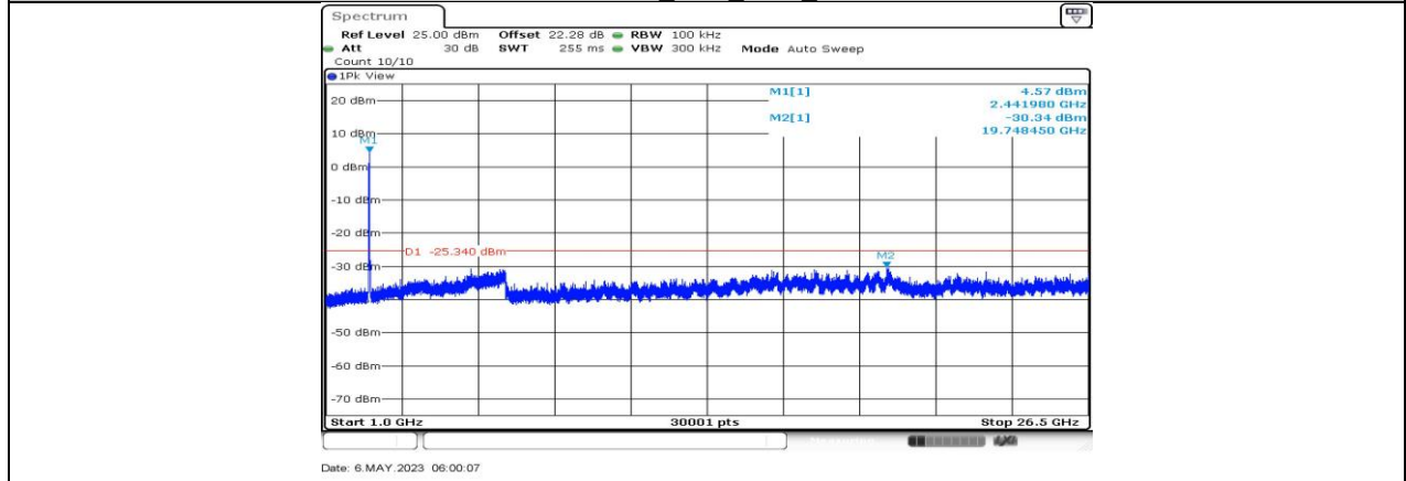
11AX40MIMO_Ant4_2447_1000-26500
