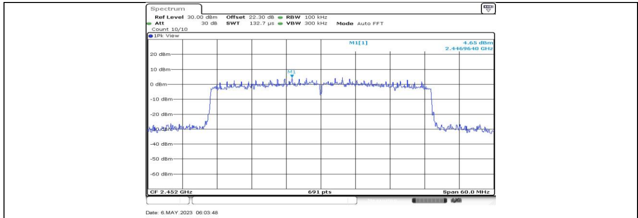
11AX40MIMO_Ant4_2452_0-Reference
