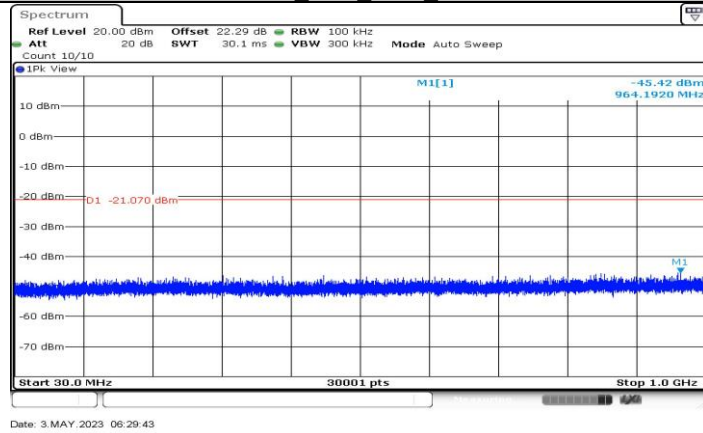
11AX20MIMO_Ant4_2417_30-1000
