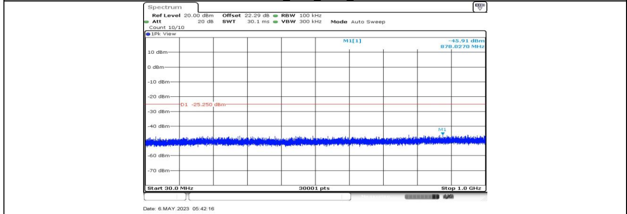
11AX40MIMO_Ant4_2422_30-1000
