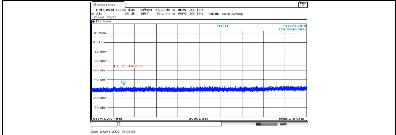
11AX40MIMO_Ant4_2452_30-1000
