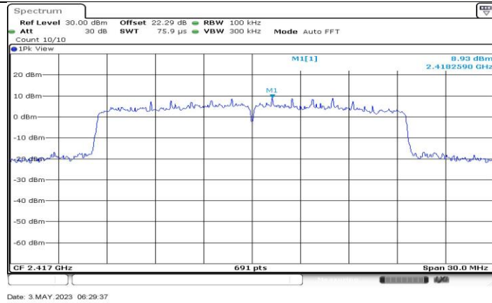
11AX20MIMO_Ant4_2417_0-Reference
