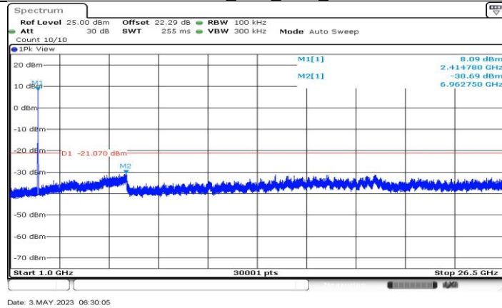
11AX20MIMO_Ant4_2417_1000-26500
