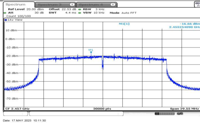
11AX20MIMO_Ant4_2457
