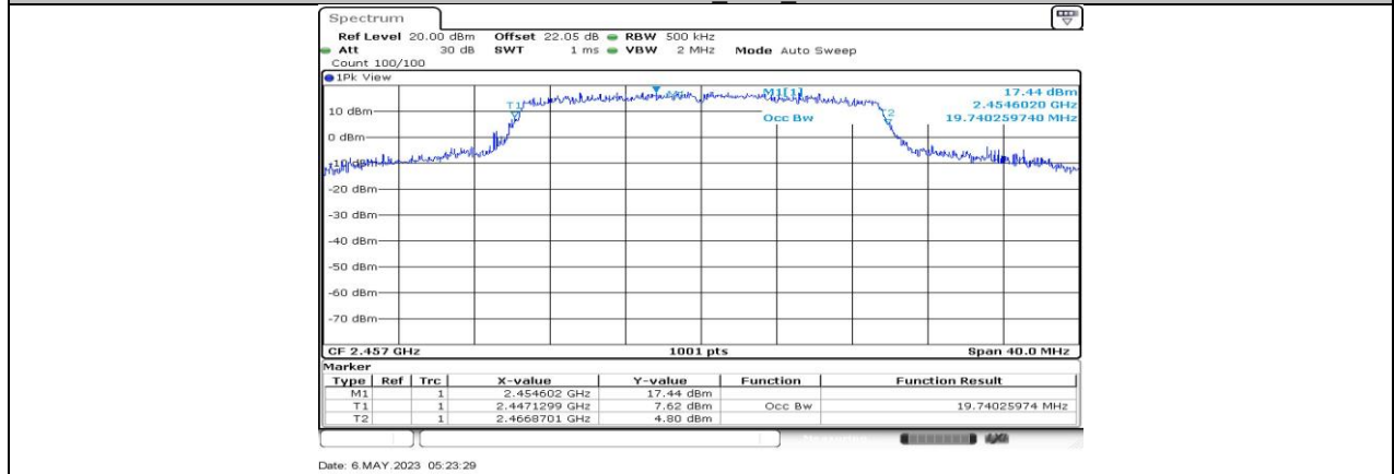
11AX20MIMO_Ant2_2457
