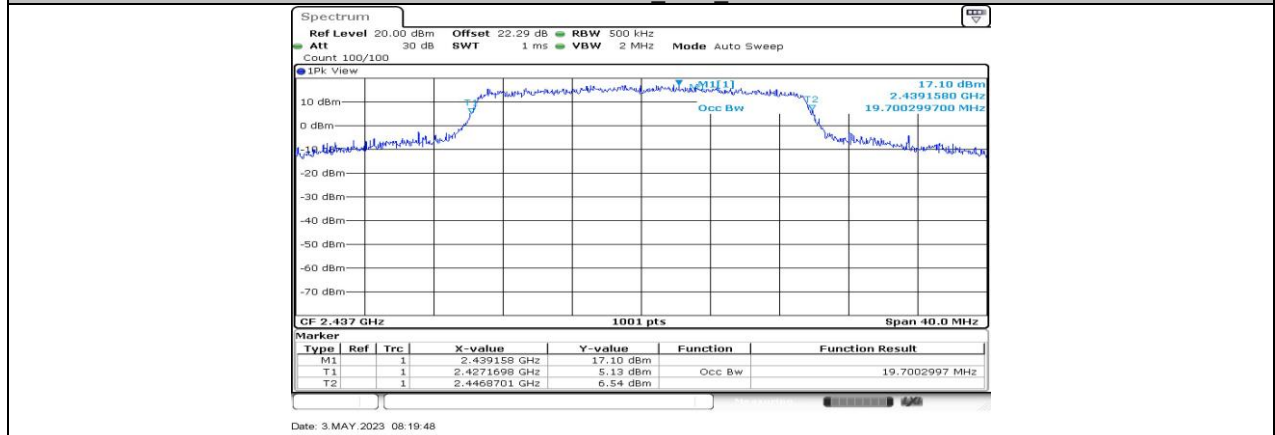
11AX20MIMO_Ant4_2437
