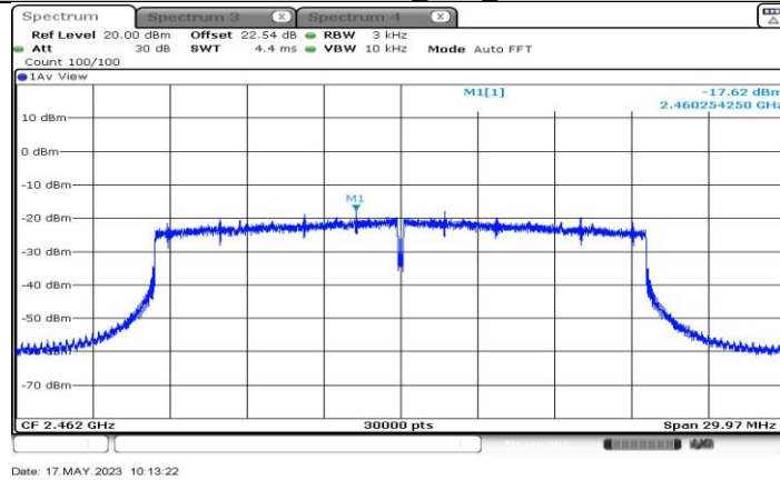
11AX20MIMO_Ant4_2462
